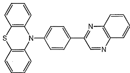
化合物 1 9
