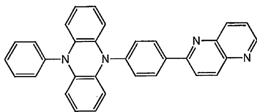
化合物 1 3
