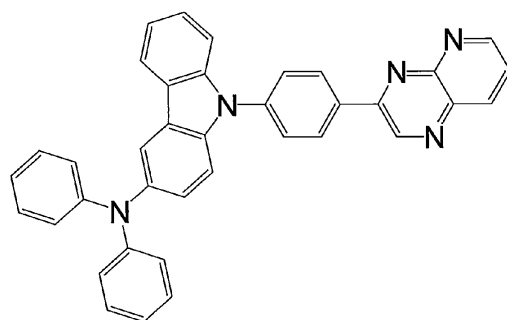
化合物 8
