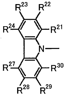
一般式 (5)
