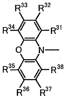
一般式 (5)
