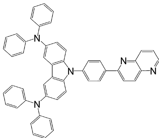
化合物 6
