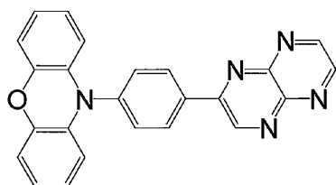
化合物 1 0
