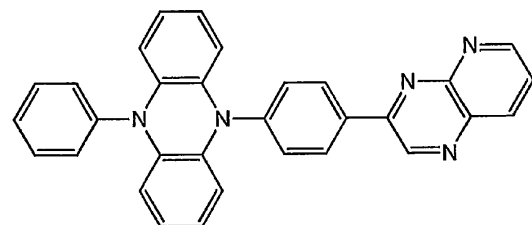
化合物 1 6
