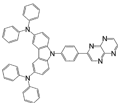
化合物 1 2
