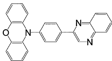
化合物 1
