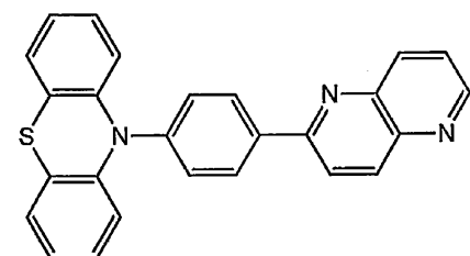
化合物 1 7
