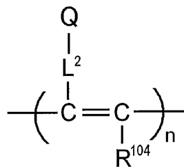
一般式 (10)
