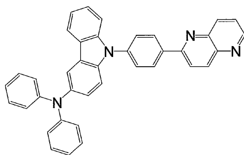
化合物 5
