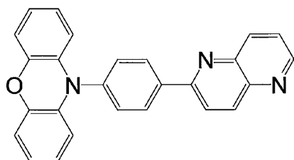
化合物 4
