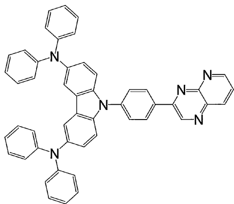
化合物 9
