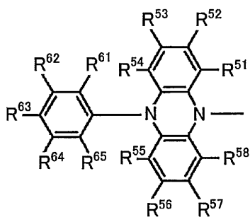
一般式 (7)
