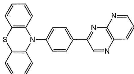
化合物 2 0
