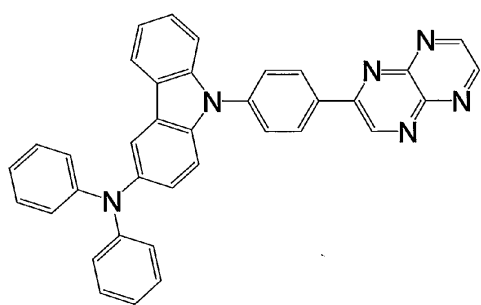
化合物 1 1
