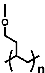
式(11)
