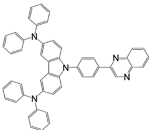
化合物 3
