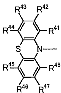
一般式 (6)
