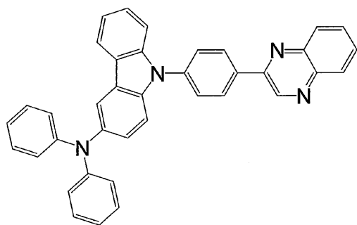
化合物 2
