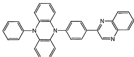
化合物 1 4
