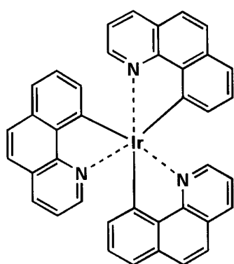
Ir-3
