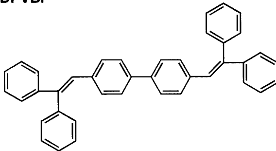
DPVBi
