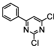
中間体 3
