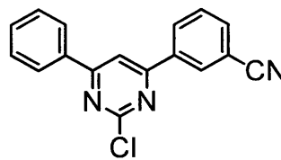
中間体 5
