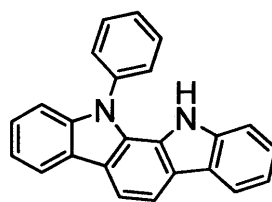
中間体 2
