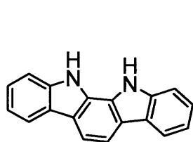
中間体 1
