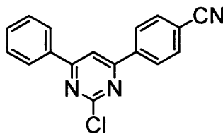
中間体 4
