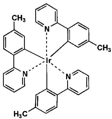
Ir-2
