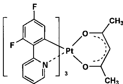
Pt-2
