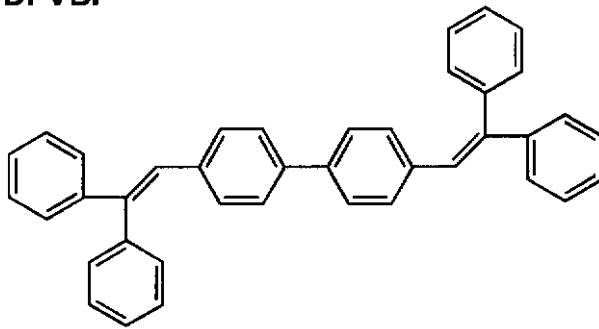
DPVBi
