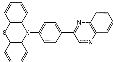
化合物 1 9
