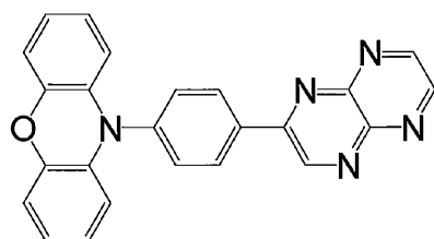
化合物 1 0
