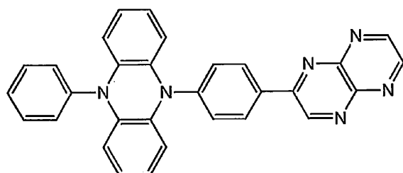
化合物 1 5
