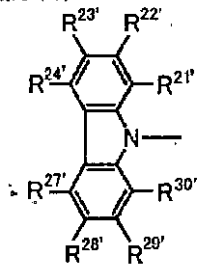
一般式 (8)
