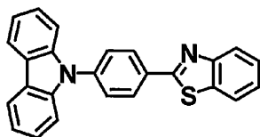
比較化合物
