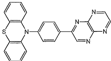
化合物 1 8
