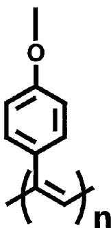
式(14)
