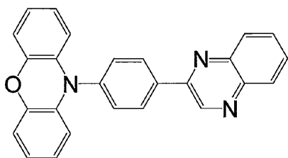
化合物 1
