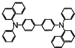
\alpha -NPD
