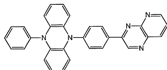
化合物 1 6
