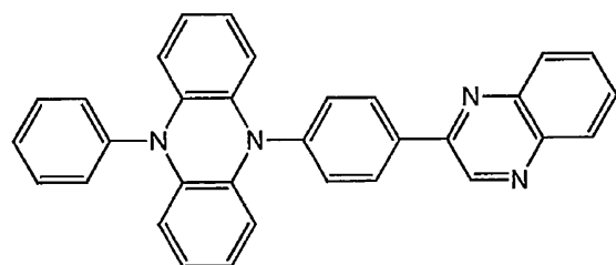
化合物 1 4
