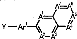
一般式(3)
