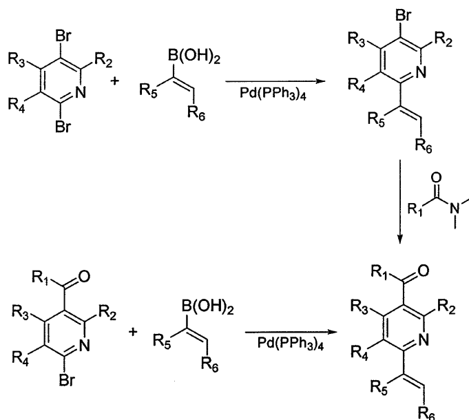
反応図式4
