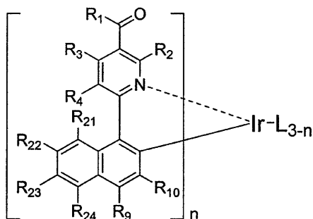
化学式7
