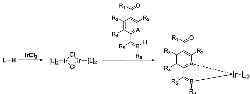
反応図式2
