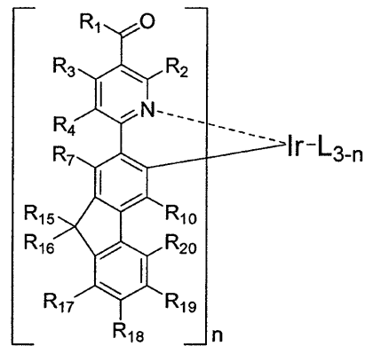
化学式5
