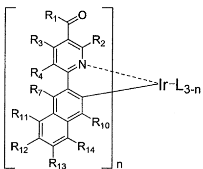
化学式4
