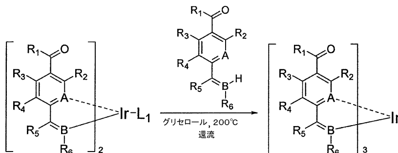
反応図式3
