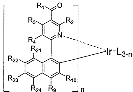
化学式7
