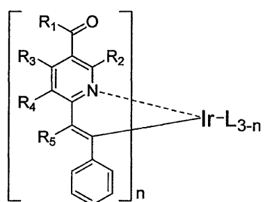
化学式3
