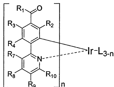
化学式7
