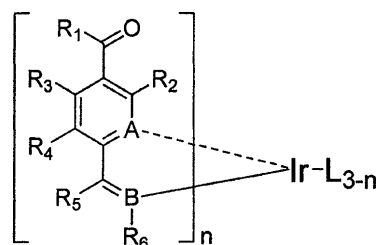
化学式 1
