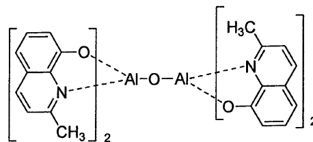
化学式10
