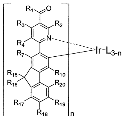
化学式5
