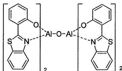
化学式9
