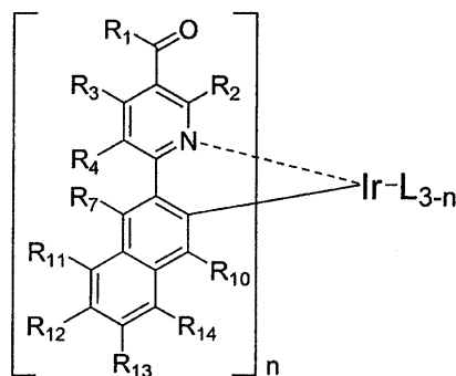
化学式4
