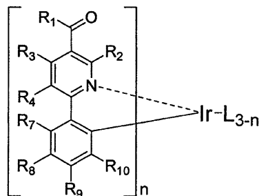
化学式4
