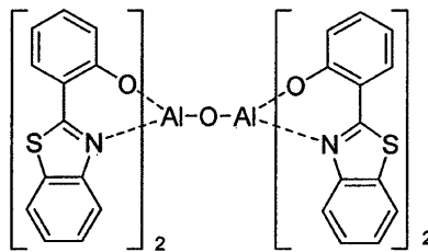
化学式9
