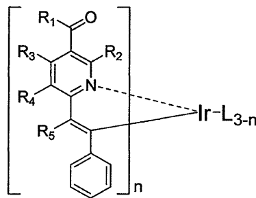
化学式3
