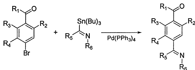
反応図式5
