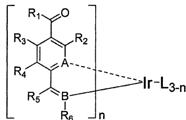
化学式1
