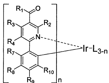
化学式4
