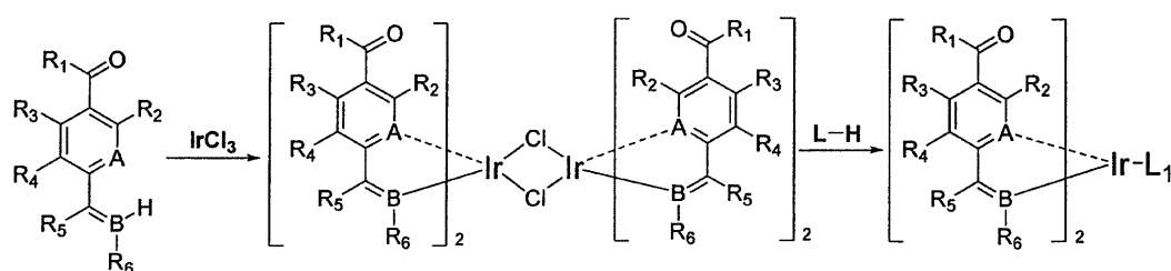
反応図式3
