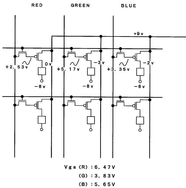
アナログ電流駆動時のバイアス例
