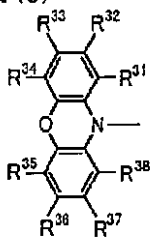
一般式 (6)
