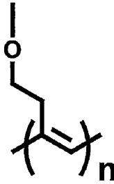
式(12)
