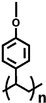
式(13)
