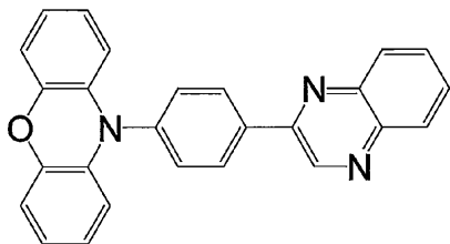
化合物 1
