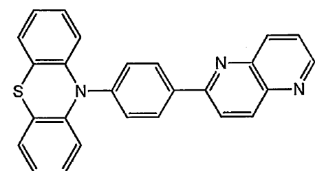
化合物 1 7
