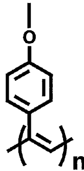
式(14)
