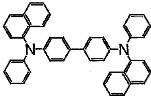
\alpha -NPD
