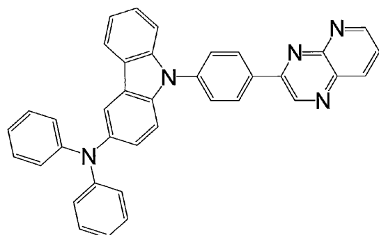
化合物 8
