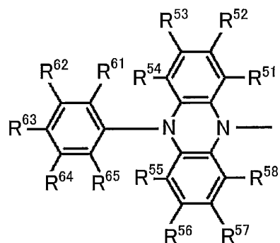
一般式 (7)
