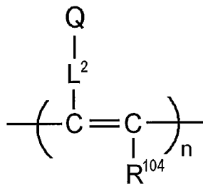
一般式 (10)
