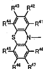
一般式 (7)
