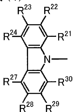
一般式 (4)
