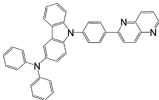
化合物 5
