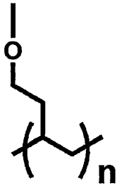
式(11)
