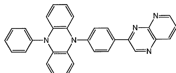
化合物 1 6
