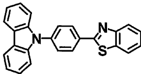
比較化合物
