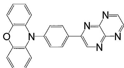
化合物 1 0
