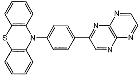
化合物 1 8
