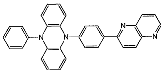
化合物 1 3
