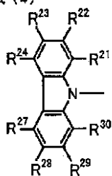
一般式 (5)
