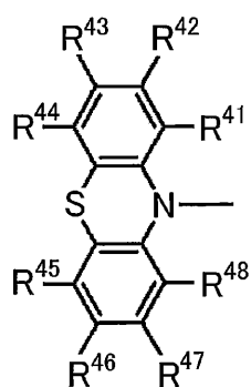
一般式 (7)
