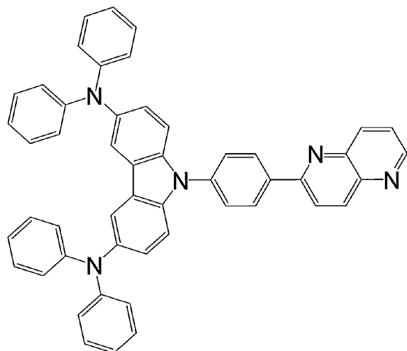
化合物 6
