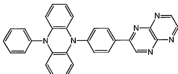
化合物 1 5
