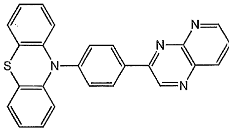
化合物 2 0
