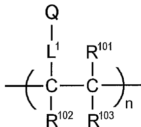
一般式 (9)
