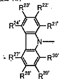
一般式 (8)
