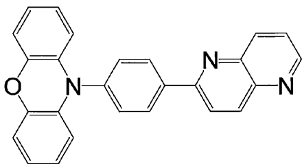
化合物 4
