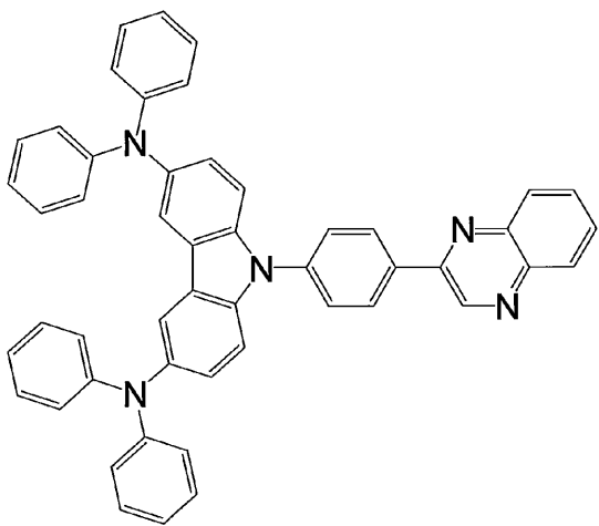
化合物 3
