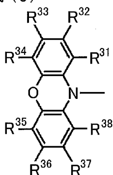
一般式 (5)
