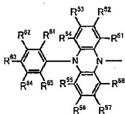
一般式 (7)
