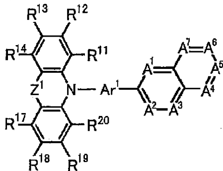
一般式(2)
