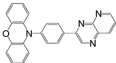
化合物 7
