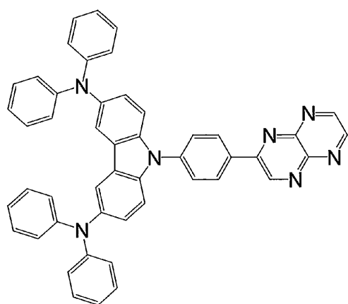
化合物 1 2
