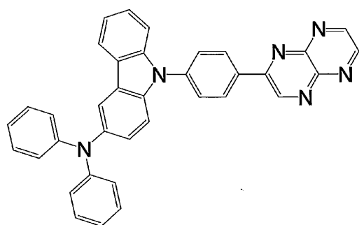
化合物 1 1
