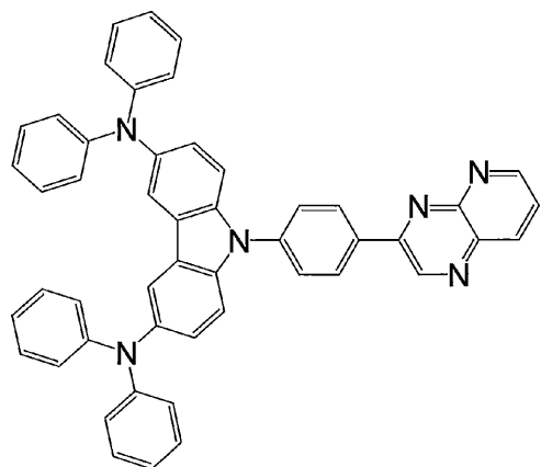
化合物 9
