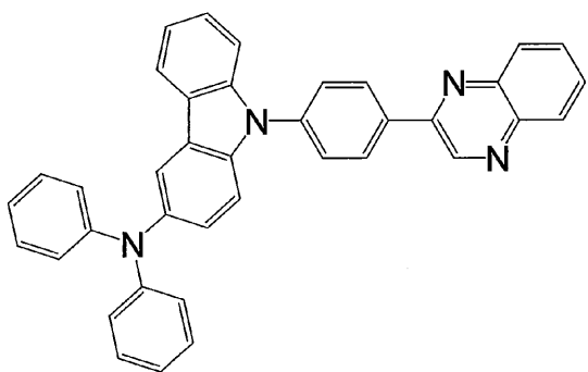
化合物 2
