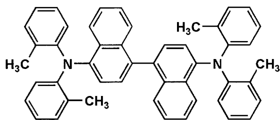
化合物H-2
