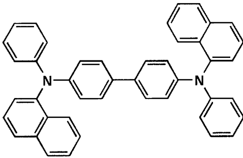
化合物H-1
