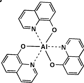
化合物E-1
