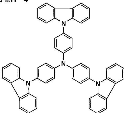
化合物H-4
