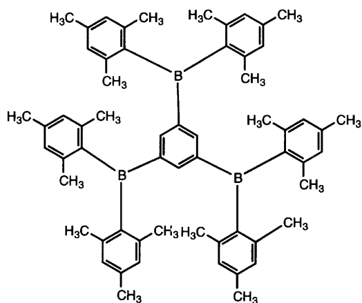
比較化合物 4
