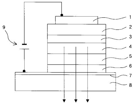
1 陰極、2 電子輸送層、3 正孔ブロック層、4 発光層 5 正孔輸送層、6 正孔注入層、7 陽極、8 基板、9 電源
