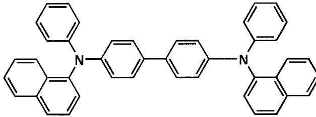
\alpha -NPD
