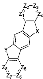
[化学式 4]
