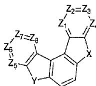
〔化学式2〕
