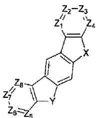
〔化学式3〕
