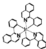
Ir(piq) 3
