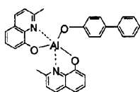
BAlq
