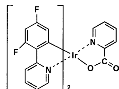
Ir-12
