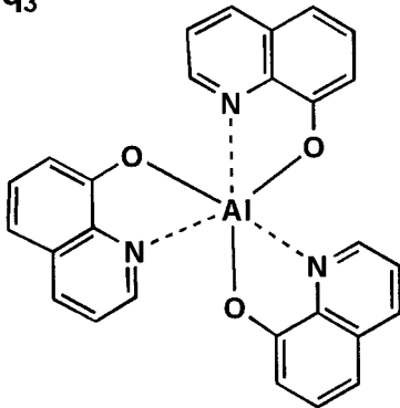
Alq 3
