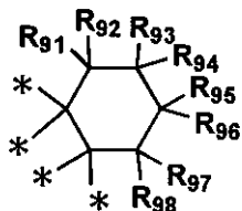
一般式(j)
