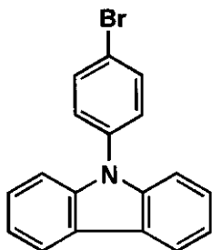
化合物(A)
