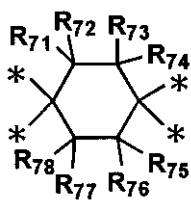
一般式(h)
