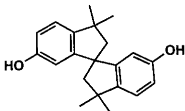
ビスフェノール
