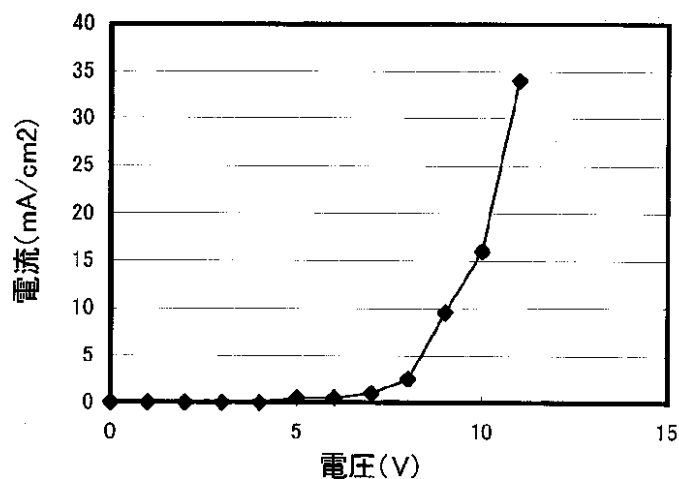
図2 電圧-電流特性
