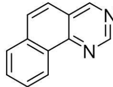
ベンゾ[h]キノリン
