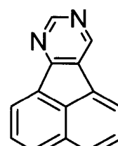
ジアザフルオランテン
