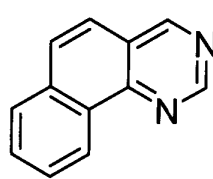
ベンゾ[h]キナゾリン
