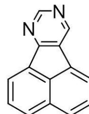
ジアザフルオランテン
