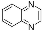
キノキサリン
