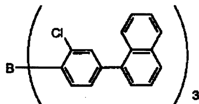
I-6
