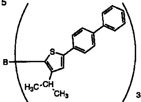
I-5
