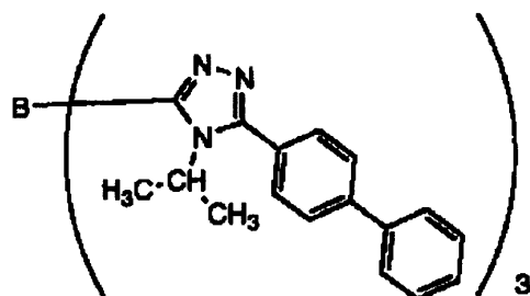
I-4
