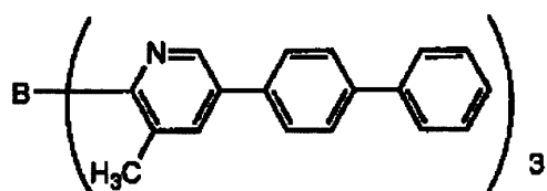
I-1
