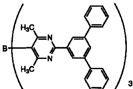
I-3
