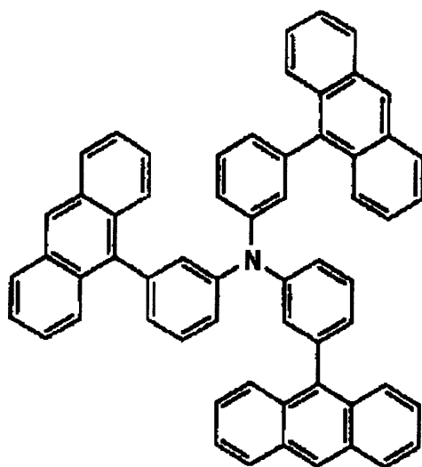
BP-5
