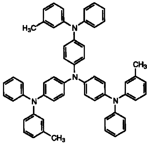
m - MTDATA
