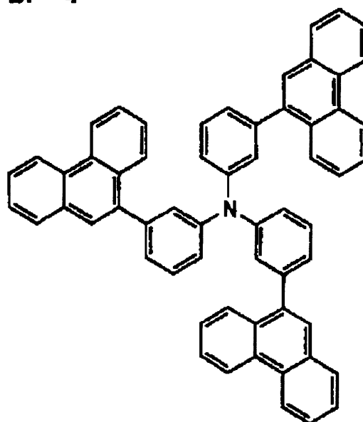
BP-6
