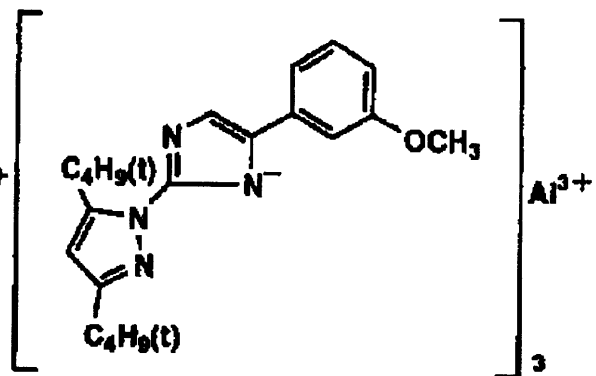
BP-26
