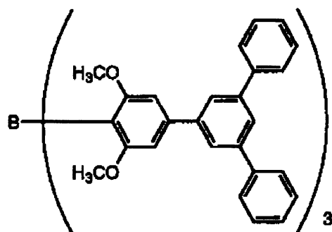
I-8
