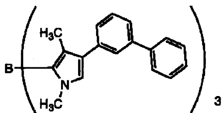
I-2
