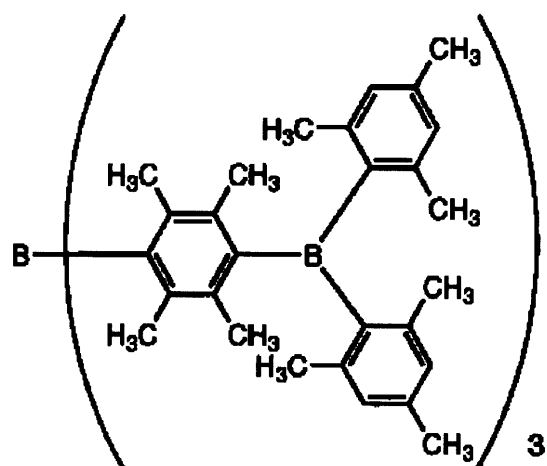
I-27
