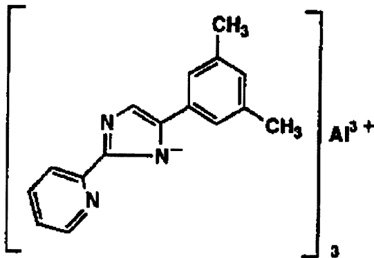
BP-25
