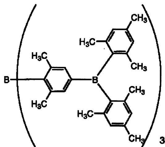
I-29
