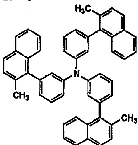
BP-3
