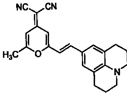
DCM2
