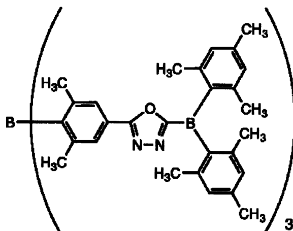
I-30
