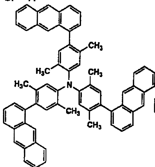
BP-11
