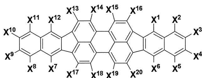
一般式 ( 1 )
