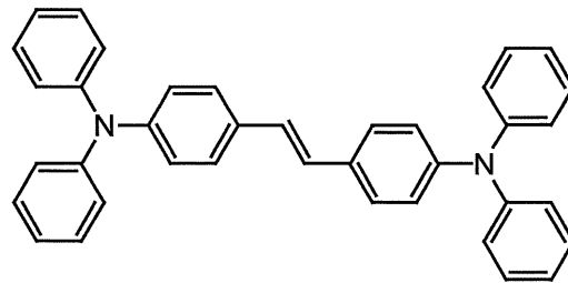
構造式(105)
