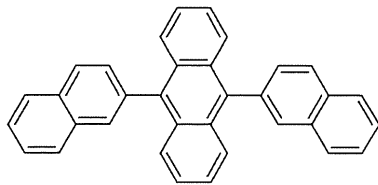
構造式(104) ADN
