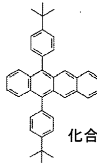
化合物(2)-2
