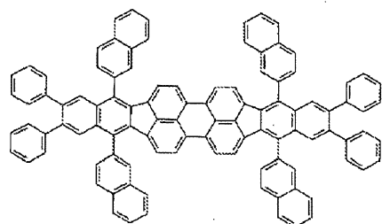
化合物(1)-5
