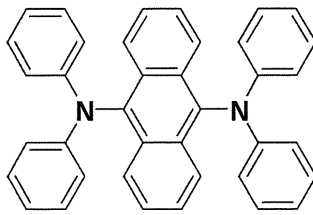
構造式(112)
