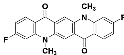
構造式(116)
