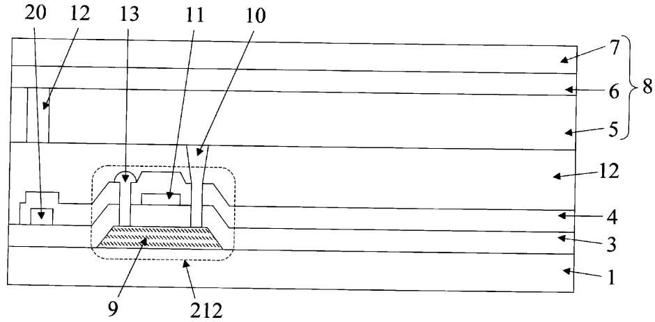
断面B-B'
