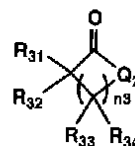
一般式(3)
