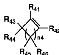
一般式(4)
