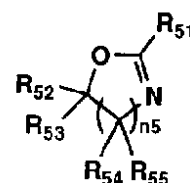
一般式(5)
