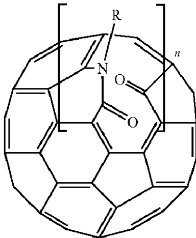
Ketolactam
