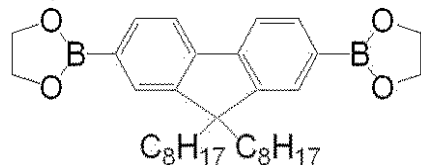
化合物A
