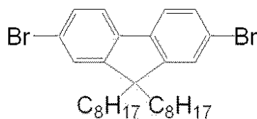
化合物B
