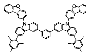
化合物 (36)
