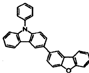
化合物 (H 6)
