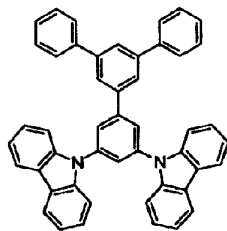
化合物（A-1）
