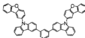
化合物 (33)
