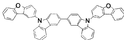
化合物 (1)
