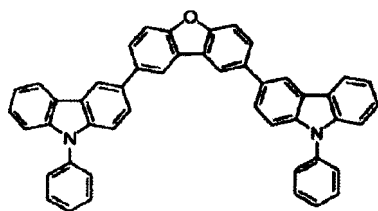
化合物 (H 4)
