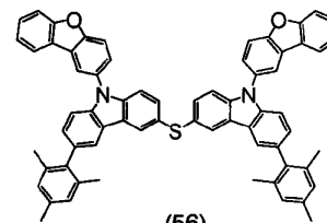
(56)
