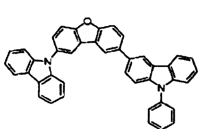
化合物 (H 5)
