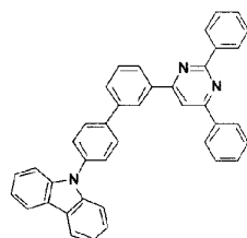
化合物 (HB)
