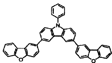
化合物 (H 1)
