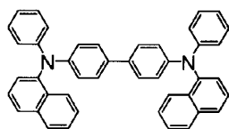
化合物 (HT)
