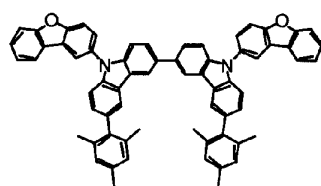
化合物 (3)
