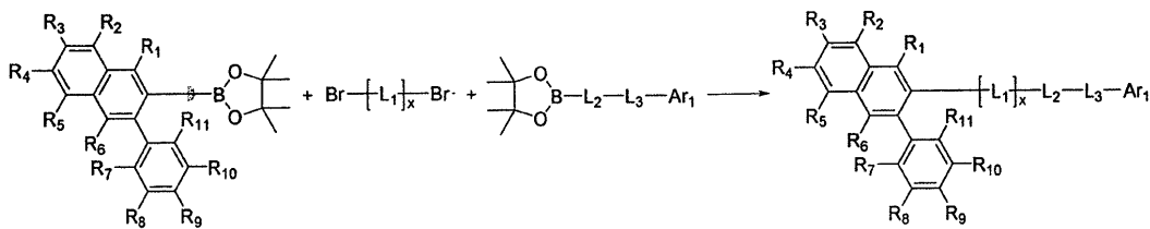
反応式2
