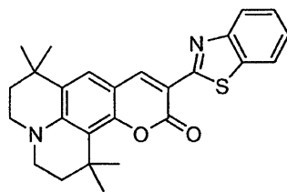
化学式3
