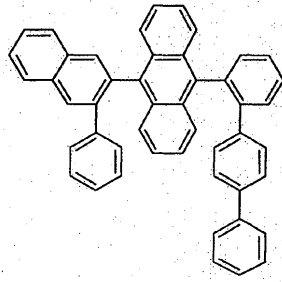
化合物705
