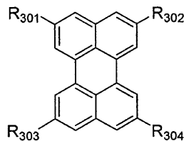
化学式 2
