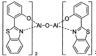
化学式9
