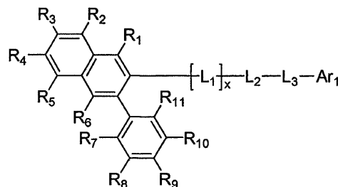
化学式1
