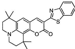
化学式3
