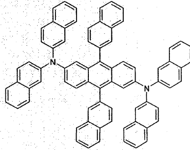
化合物E
