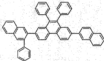
化合物218
