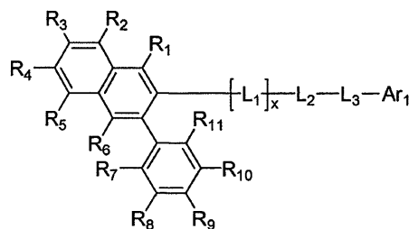
化学式 1
