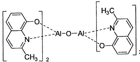
化学式10
