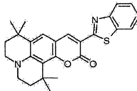
C545T
