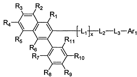
化学式 1
