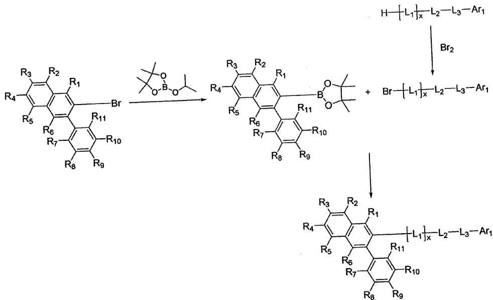
反応式1
