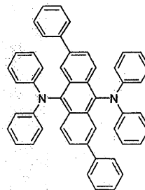
化合物A
