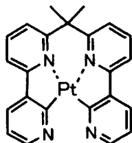
化合物 (84)
