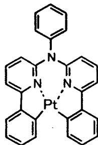
化合物 (82)
