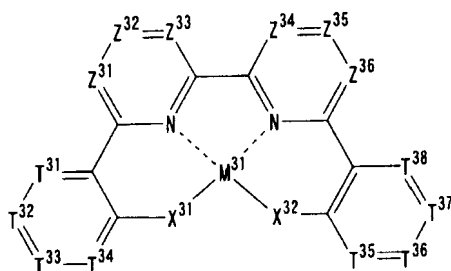
一般式(3)
