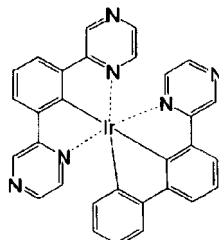
化合物 (125)
