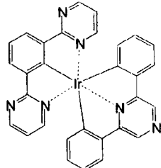
化合物 (127)
