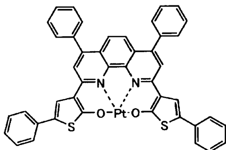
化合物 (205)
