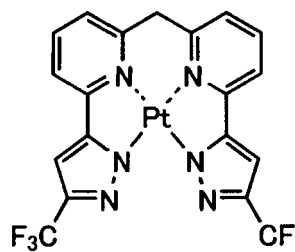
化合物 (222)
