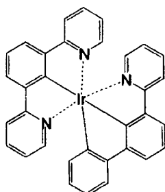
化合物 (109)
