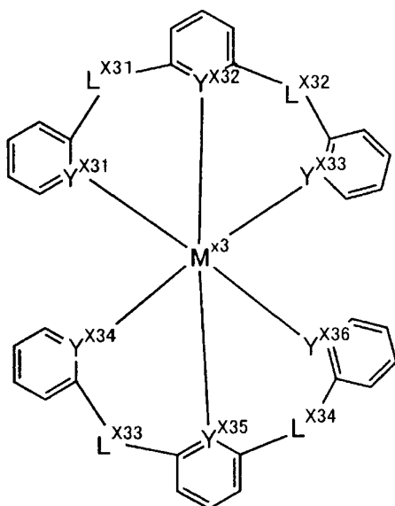
一般式 (X3)
