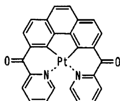
化合物(36)
