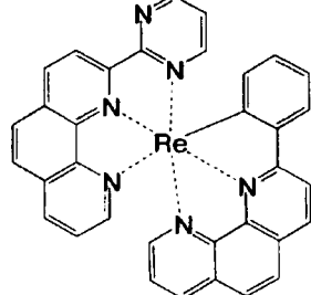
化合物 (132)
