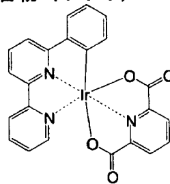
化合物 (115)
