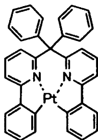
化合物 (78)
