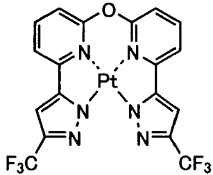
化合物 (223)
