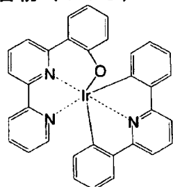
化合物 (116)
