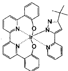
化合物 (118)
