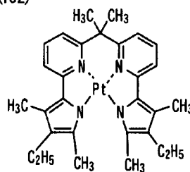
化合物(152)
