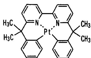
化合物(47)
