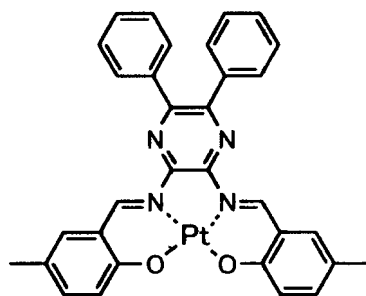
化合物 (94)
