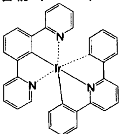
化合物 (110)
