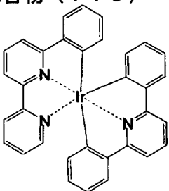
化合物 (111)
