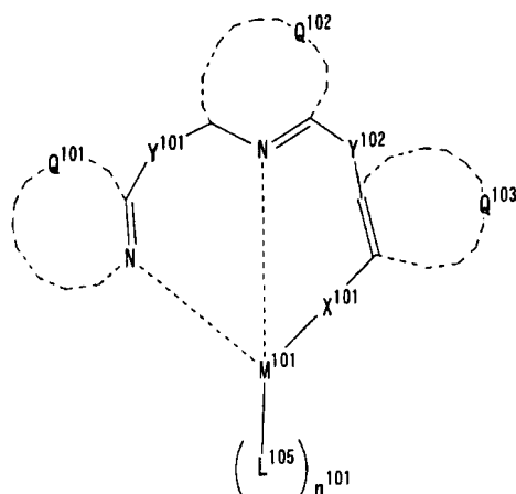
一般式(14)
