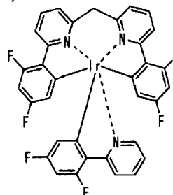
化合物(152)
