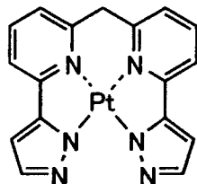
化合物 (219)
