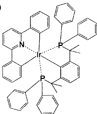
化合物 (171)
