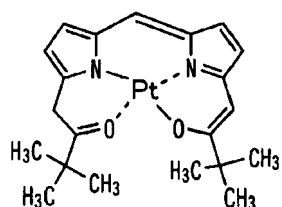
化合物(28)
