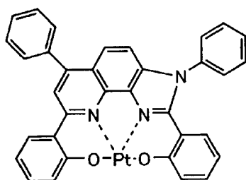
化合物 (201)
