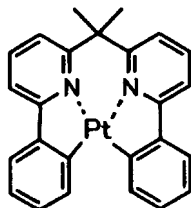
化合物 (79)
