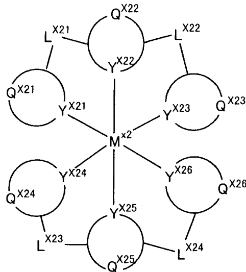
一般式 (X2)
