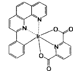
化合物 (121)
