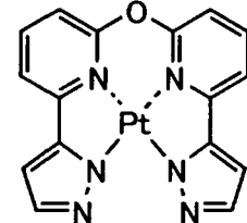
化合物 (220)
