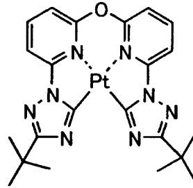
化合物 (217)
