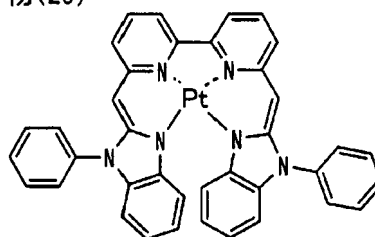
化合物(29)
