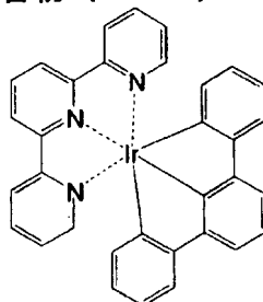
化合物 (112)
