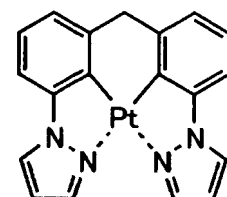
化合物 (228)
