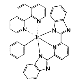
化合物 (122)
