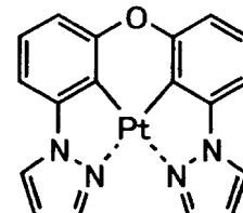
化合物 (229)
