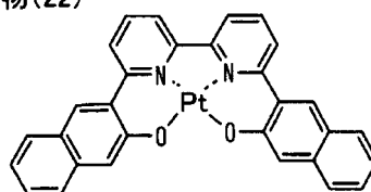
化合物(22)
