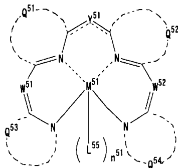
一般式(5)
