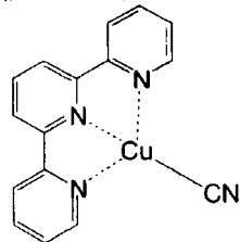
化合物 (136)
