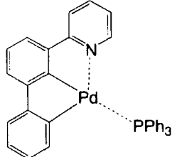
化合物 (137)
