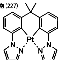
化合物 (230)
