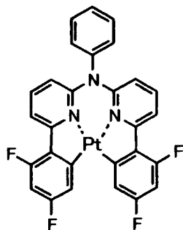
化合物 (81)
