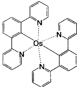
化合物 (132)
