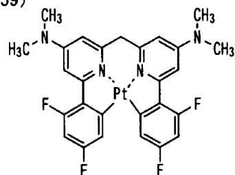
化合物(60)
