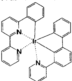
化合物 (112)
