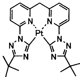
化合物 (216)
