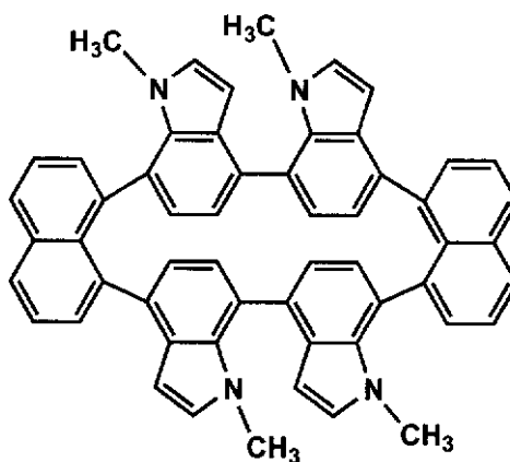
化合物(12)
