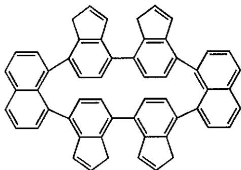
化合物(5)
