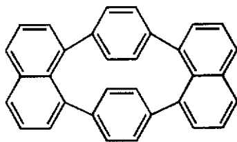
化合物(1)
