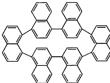
化合物(4)
