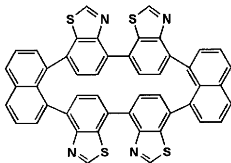
化合物(7)
