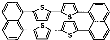
化合物(9)
