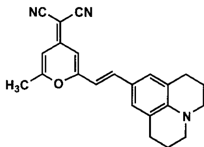
DCM-2
