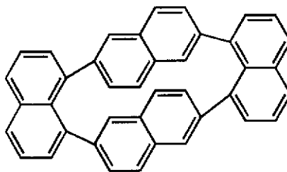
化合物(4)
