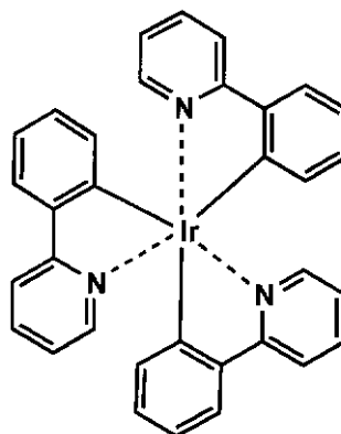
Ir-1
