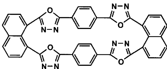
化合物(15)
