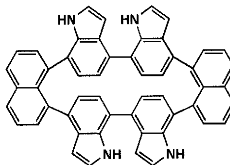
化合物(6)
