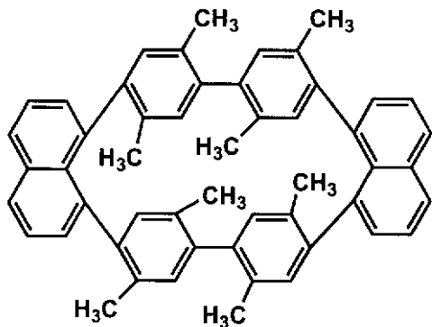
化合物(11)
