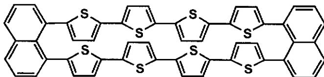
化合物(15)
