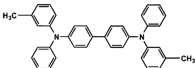
TPD
