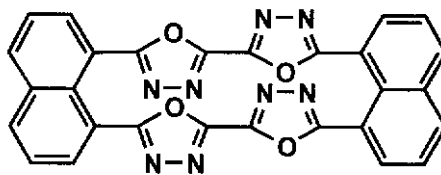
化合物(10)
