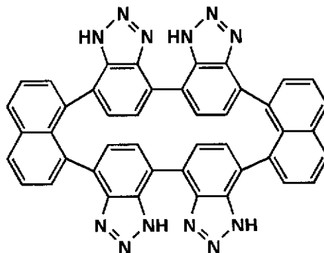
化合物(8)
