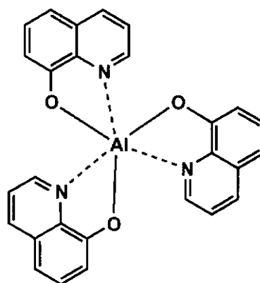
Alq 3
