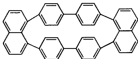
化合物(3)
