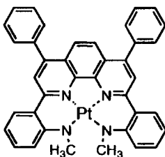
化合物 (73)
