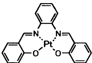
化合物 (88)
