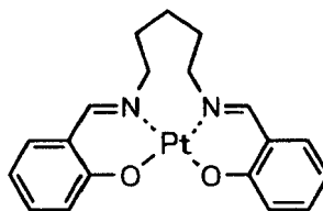
化合物 (96)
