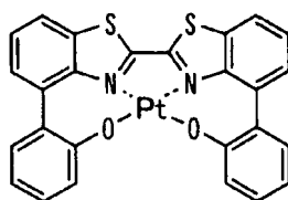
化合物(28)
