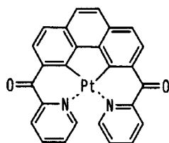
化合物(36)
