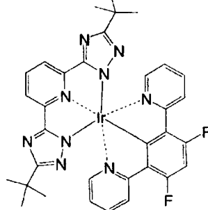
化合物 ( 1 0 7 )
