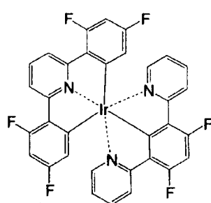
化合物 ( 1 0 4 )
