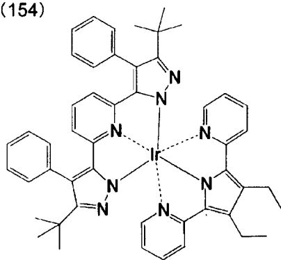
化合物(154)
