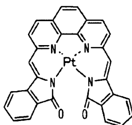
化合物(25)
