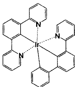
化合物 (109)
