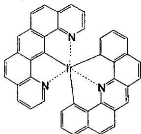
化合物 ( 9 9 )
