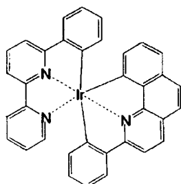
化合物 ( 1 0 2 )
