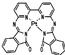
化合物(27)
