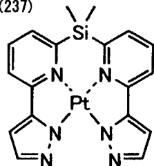
化合物 (237)
