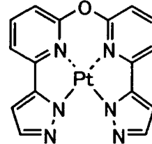
化合物 (220)
