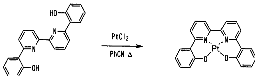
化合物(1)
