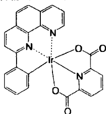
化合物 (122)
