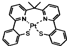
化合物 (69)
