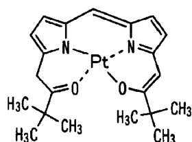
化合物(28)
