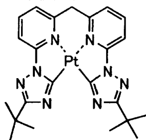
化合物 (216)
