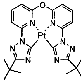
化合物 (217)
