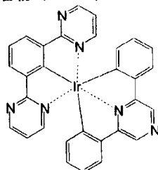
化合物 (127)
