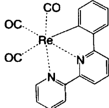
化合物 (131)
