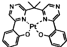
化合物 (67)
