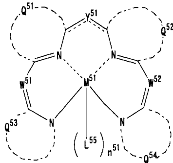
一般式(5)
