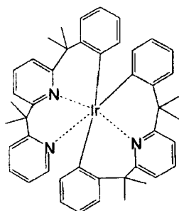
化合物 ( 1 0 2 )
