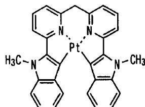
化合物(53)
