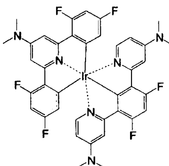
化合物 ( 1 0 5 )
