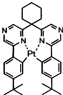
化合物 (81)
