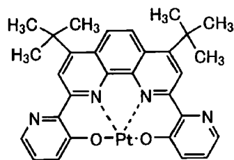
化合物 (208)
