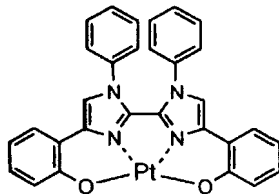
化合物 (75)
