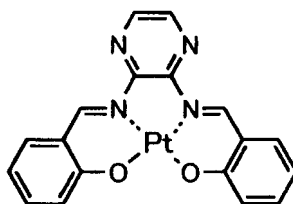
化合物 (93)
