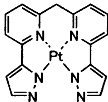
化合物 (219)
