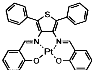
化合物 (91)
