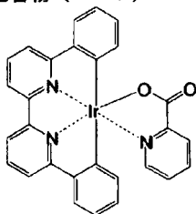
化合物 (120)
