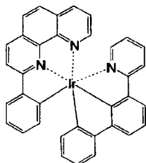
化合物 (121)
