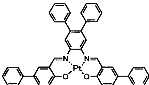
化合物 (89)
