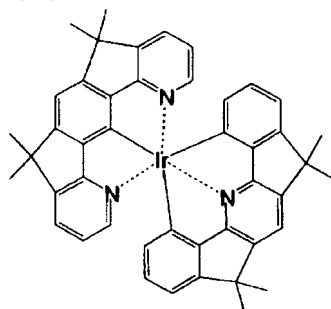
化合物 ( 1 0 0 )
