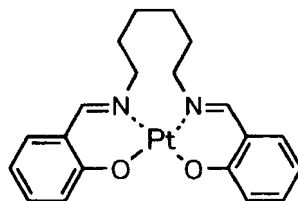
化合物 (97)
