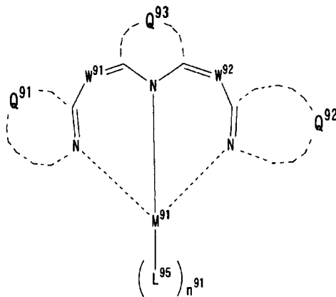
一般式(13)
