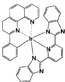
化合物 (122)
