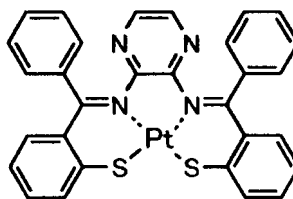
化合物 (95)
