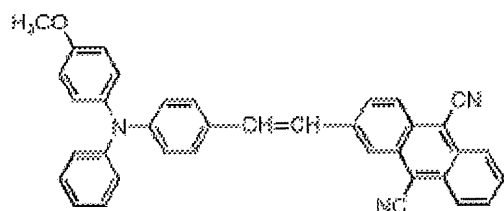
化合物(6)-11
