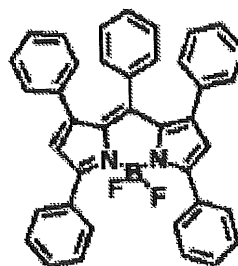
化合物(4)-22
