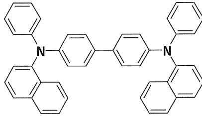
構造式(102) \alpha -NPD
