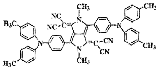
化合物(3)-12
