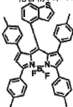
化合物(4)-60
