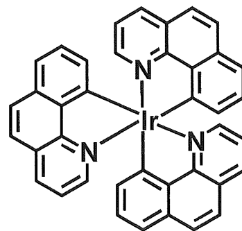
構造式(108)
