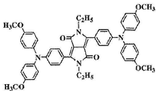
化合物(3)-5
