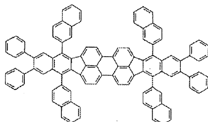
化合物(2)-5
