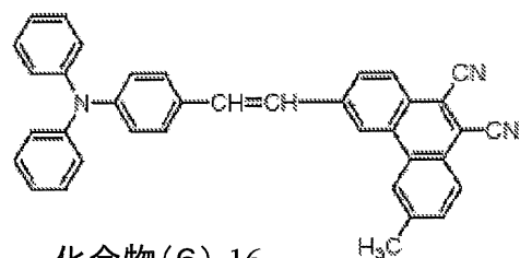
化合物(6)-16
