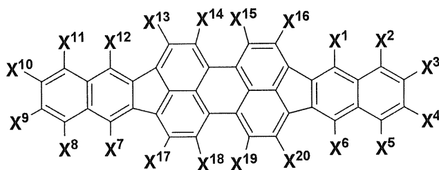
一般式 (2)
