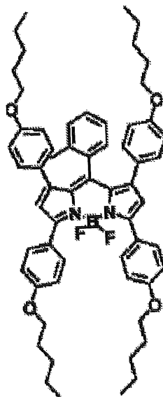
化合物(4)-39
