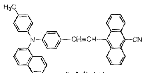
化合物(6)-15
