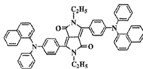
化合物(3)-8
