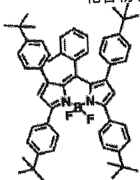
化合物(4)-36
