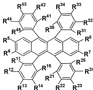
一般式(1a)
