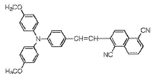
化合物(6)-8
