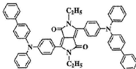
化合物(3)-6
