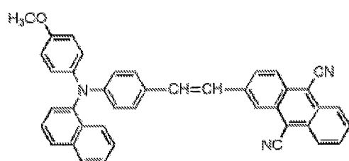
化合物(6)-13
