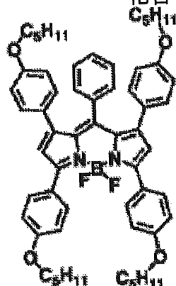
化合物(4)-29
