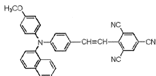
化合物(6)-5
