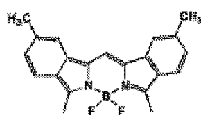
化合物(4)-7
