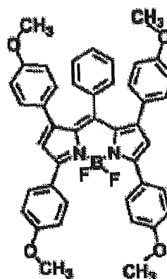
化合物(4)-28
