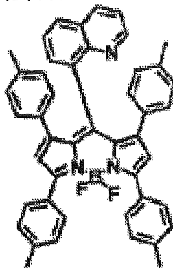
化合物(4)-55
