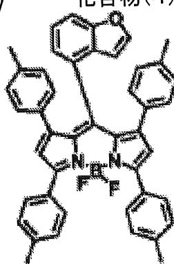
化合物(4)-58
