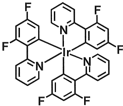
構造式(111)
