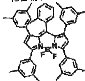
化合物(4)-35
