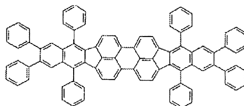
化合物(2)-4
