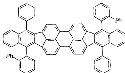
化合物(2)-7
