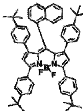
化合物(4)-66
