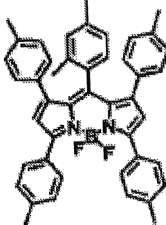
化合物(4)-45
