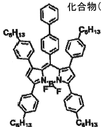
化合物(4)-26
