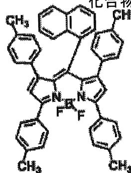
化合物(4)-30
