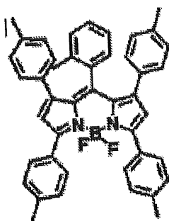
化合物(4)-36
