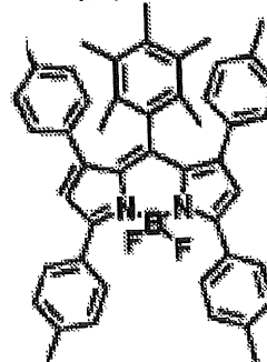
化合物(4)-46
