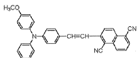
化合物(6)-7
