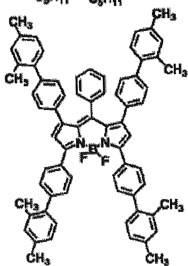
化合物(4)-31
