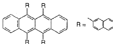
化合物(1)-2
