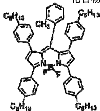
化合物(4)-23
