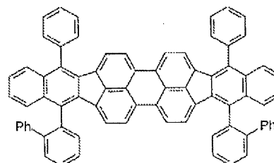
化合物(2)-8
