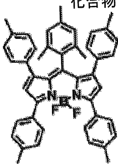
化合物(4)-44
