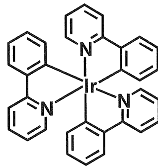
構造式(105) \text{Ir}(\text{ppy})_3
