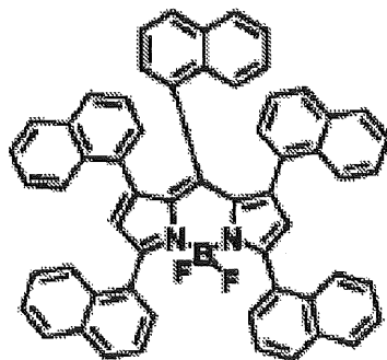
化合物(4)-67
