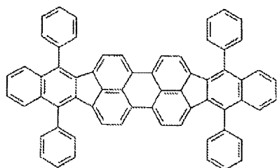
化合物(2)-1
