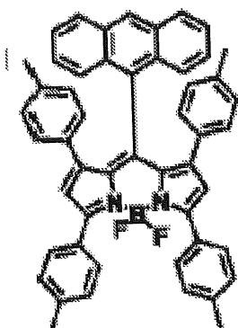
化合物(4)-49
