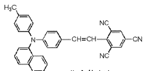
化合物(6)-6
