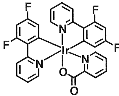
構造式(110)
