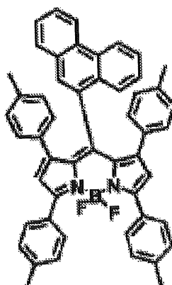
化合物(4)-52
