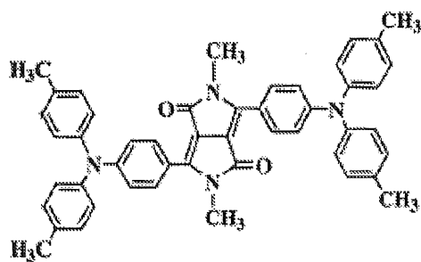
化合物(3)-2
