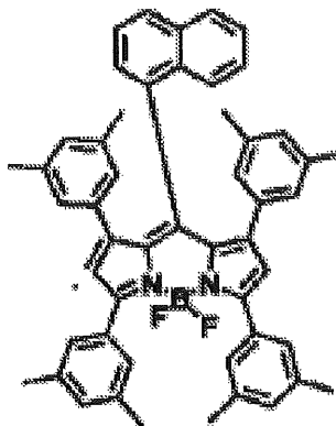
化合物(4)-66
