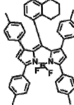
化合物(4)-62
