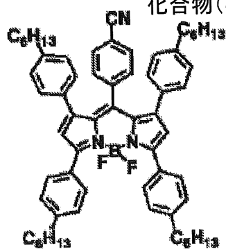
化合物(4)-25
