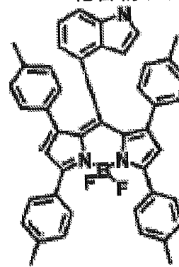
化合物(4)-59
