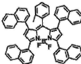
化合物(4)-43
