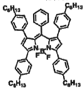
化合物(4)-21
