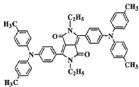
化合物(3)-4
