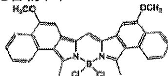
化合物(4)-9
