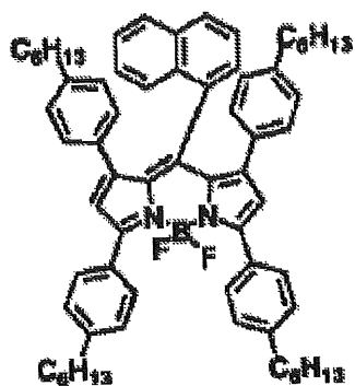
化合物(4)-29
