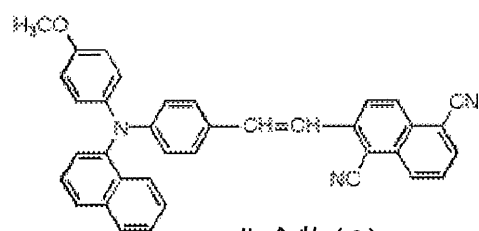
化合物(6)-9
