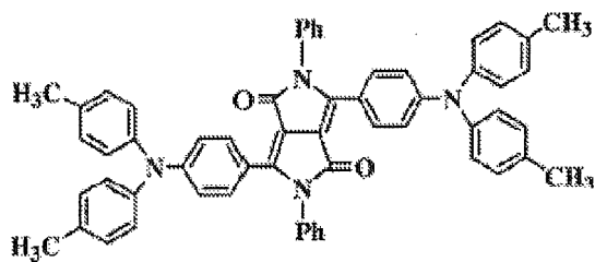
化合物(3)-9
