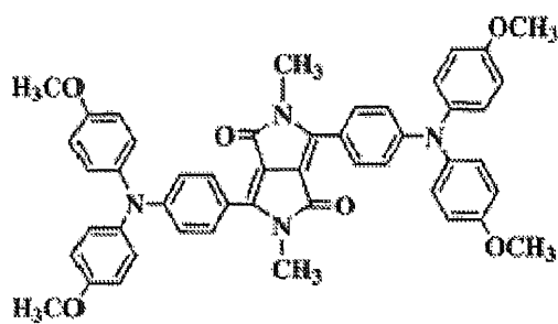
化合物(3)-3
