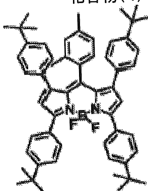
化合物(4)-47
