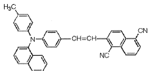
化合物(6)-10
