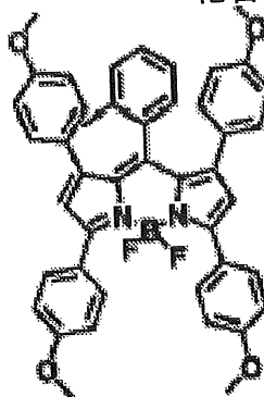
化合物(4)-41
