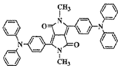
化合物(3)-1
