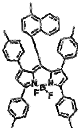
化合物(4)-57
