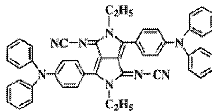
化合物(3)-14
