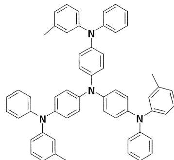
構造式(101) MADATA
