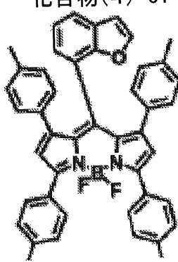
化合物(4)-61
