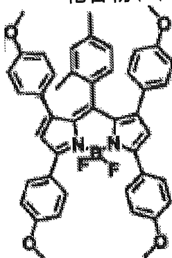
化合物(4)-48
