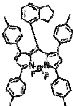
化合物(4)-63
