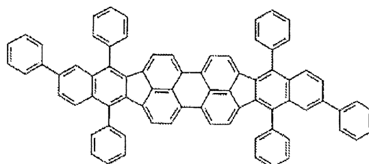
化合物(2)-2
