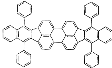
構造式(103) ペリレン誘導体
