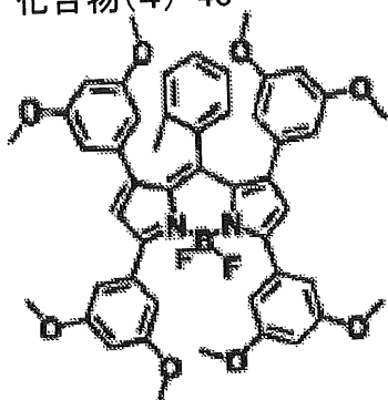
化合物(4)-42
