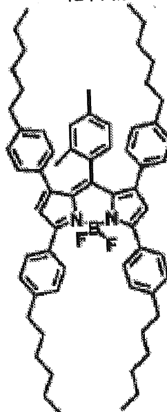
化合物(4)-50
