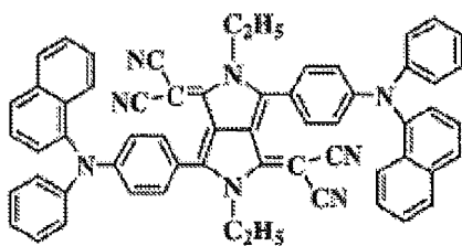
化合物(3)-13
