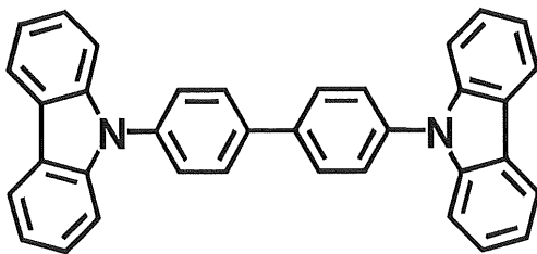
構造式(104) CBP
