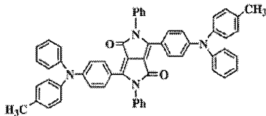
化合物(3)-10
