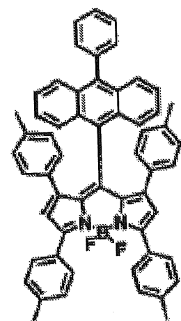
化合物(4)-51
