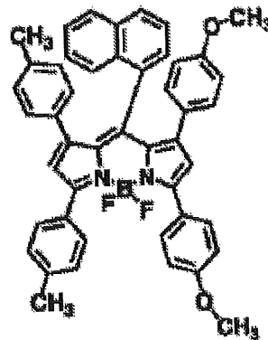
化合物(4)-32
