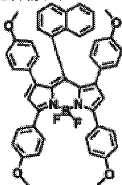
化合物(4)-65
