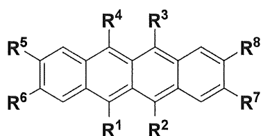
一般式(1)
