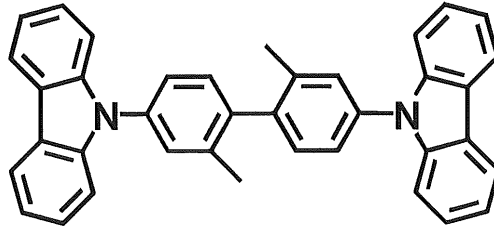
構造式(109)
