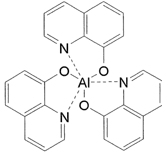
構造式(106) Alq3
