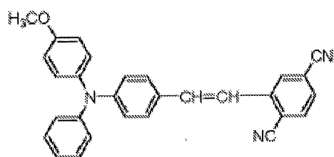
化合物(6)-1
