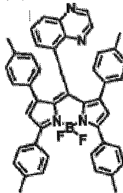
化合物(4)-56
