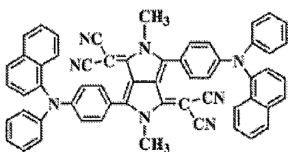
化合物(3)-11
