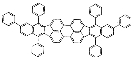
化合物(2)-3
