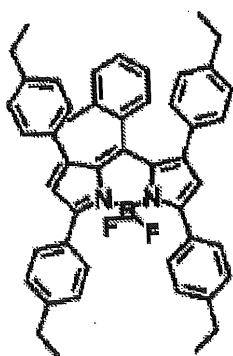
化合物(4)-38
