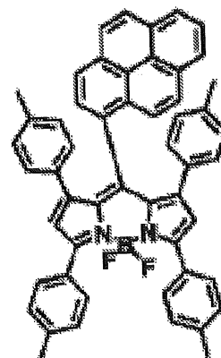
化合物(4)-53
