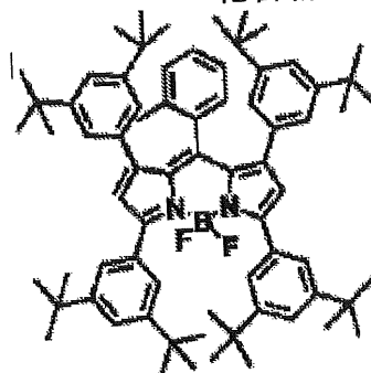
化合物(4)-37
