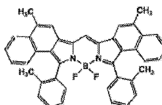
化合物(4)-14
