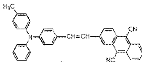
化合物(6)-12
