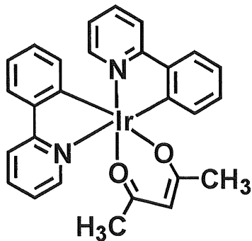
構造式(107)
