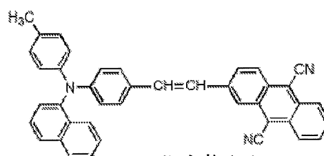
化合物(6)-14
