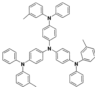
(101) m-MTDATA
