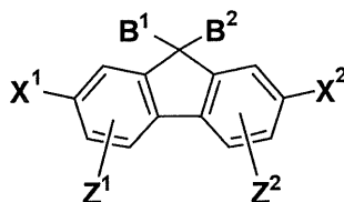
一般式(2)
