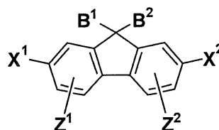
一般式(2)
