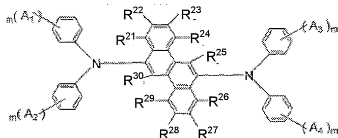
一般式(4)
