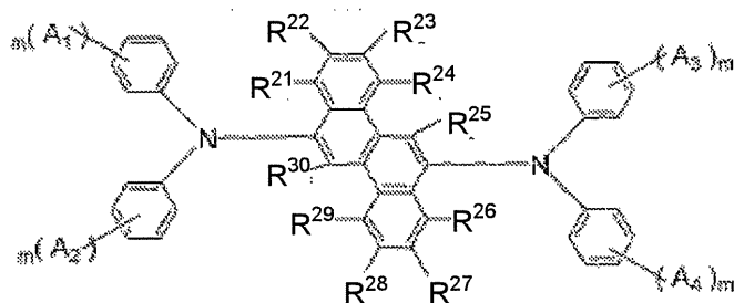
一般式(4)
