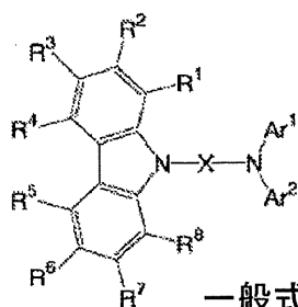
一般式(1)
