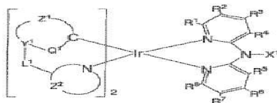
一般式(1)
