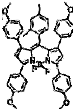
化合物(5)-48
