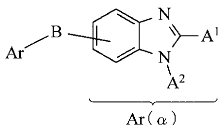
一般式 (1)
