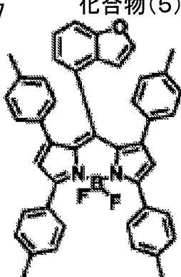
化合物(5)-58
