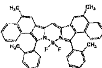
化合物(5)-14
