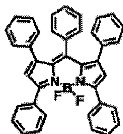
化合物(5)-22
