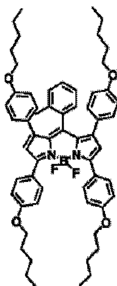
化合物(5)-39
