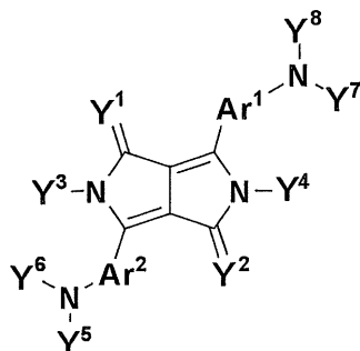
一般式(4)
