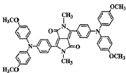
化合物(4)-3
