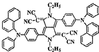
化合物(4)-13
