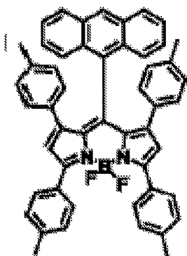
化合物(5)-49
