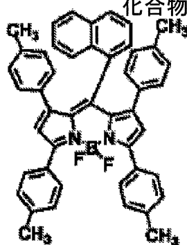
化合物(5)-30
