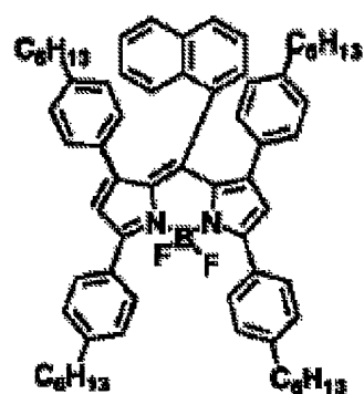
化合物(5)-29
