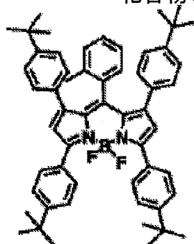
化合物(5)-36
