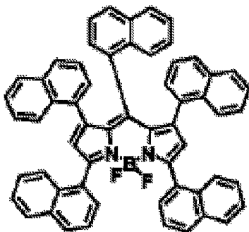
化合物(5)-67
