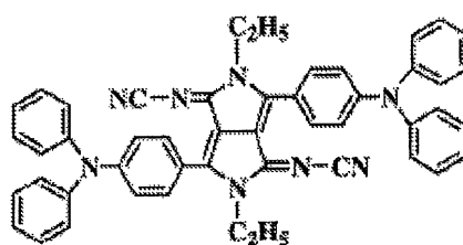
化合物(4)-14
