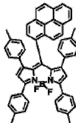
化合物(5)-53
