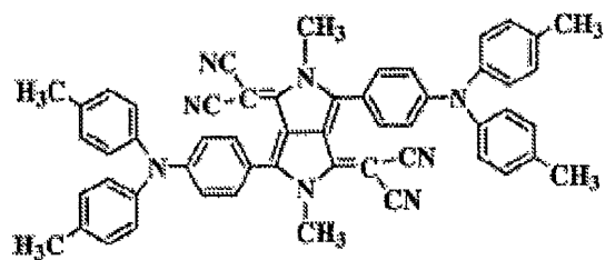
化合物(4)-12
