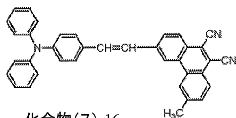
化合物(7)-16
