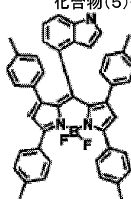
化合物(5)-59
