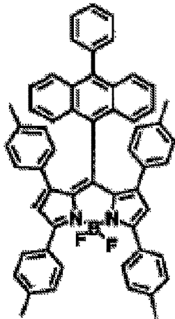
化合物(5)-51
