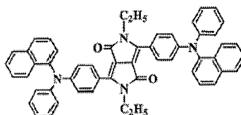
化合物(4)-8
