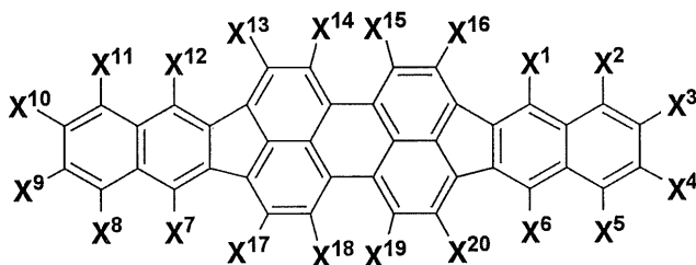
一般式 (3)
