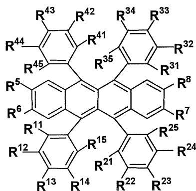
一般式(2a)
