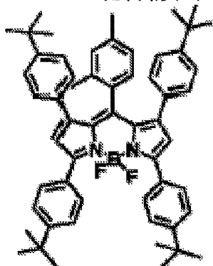
化合物(5)-47
