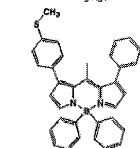
化合物(5)-4
