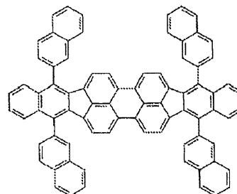
化合物(3)-6
