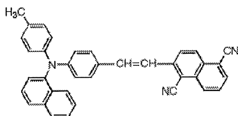
化合物(7)-10
