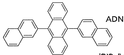
構造式(104)
