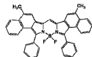
化合物(5)-13
