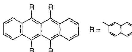
化合物(2)-2
