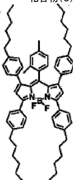
化合物(5)-50
