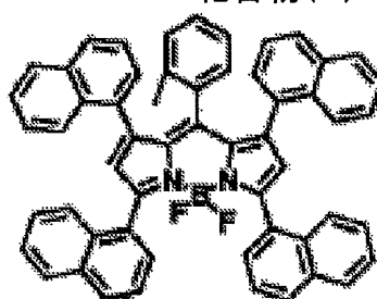
化合物(5)-43
