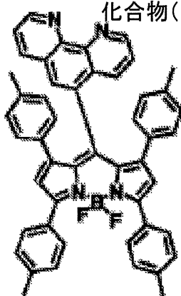
化合物(5)-60
