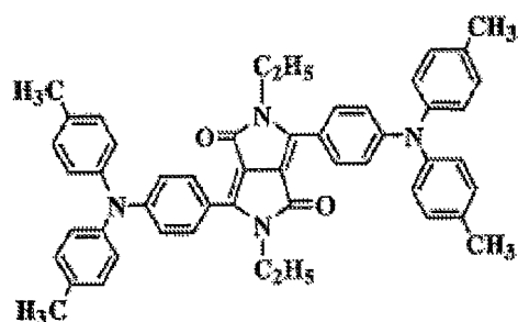
化合物(4)-4
