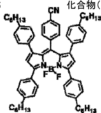
化合物(5)-25
