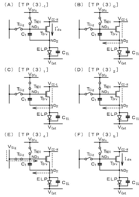
【図 10】 [実施例 3 : 3 Tr / 1 C 駆動回路]
