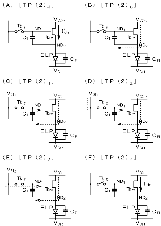
【図5】 [実施例1：2Tr／1C駆動回路]
