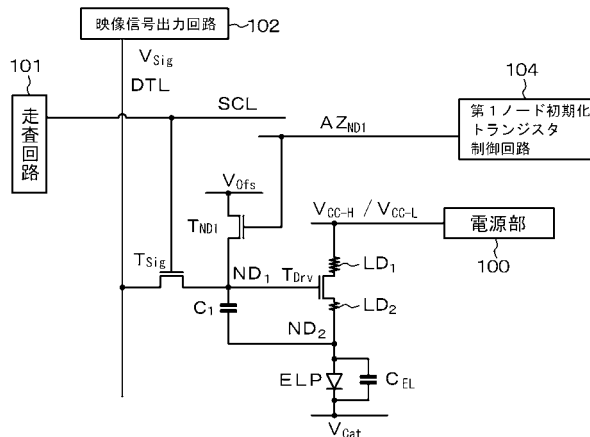
【図 1 1】 [実施例 4 : 実施例 3 の変形例]
