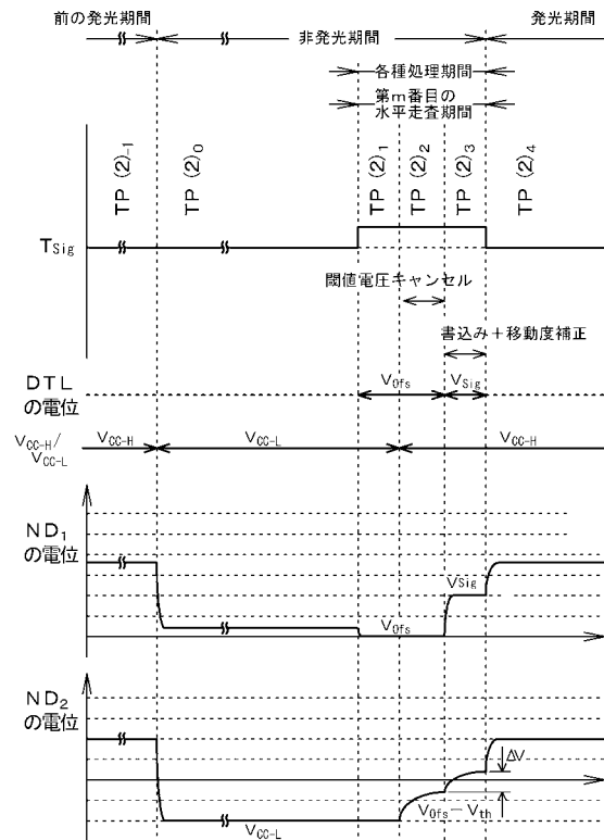
【図4】 [実施例1：2Tr／1C駆動回路]
