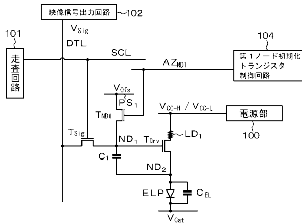
【図 7】 [実施例 3 : 3 Tr / 1 C 駆動回路]
