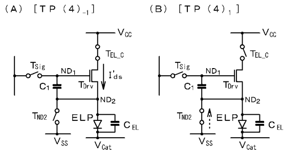
【図 1 2】 [4 Tr / 1 C 駆動回路]
