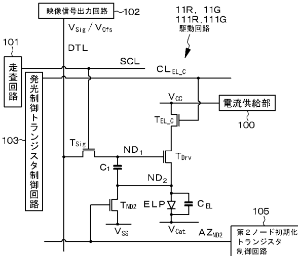
【図 9】 [4 Tr / 1 C 駆動回路]
