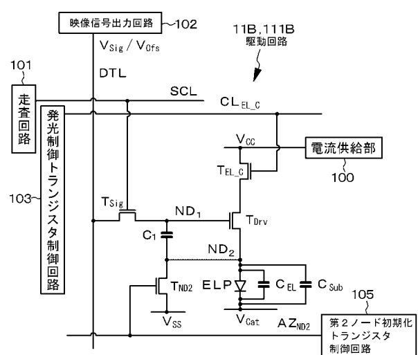
【図 8】 [4 Tr / 1 C 駆動回路]
