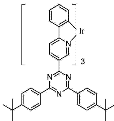
比较发射体 2
