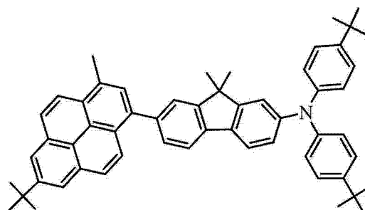
化合物 13
