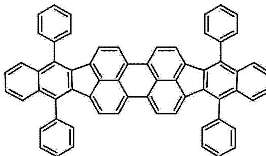
化合物 5
