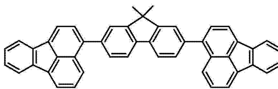
化合物 7
