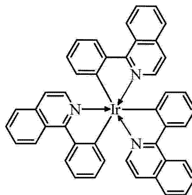
化合物 11
