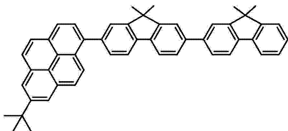
化合物 6
