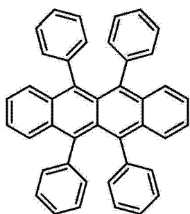
化合物 4
