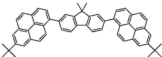
[0103] 化合物 12
