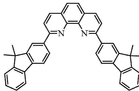
化合物 9
