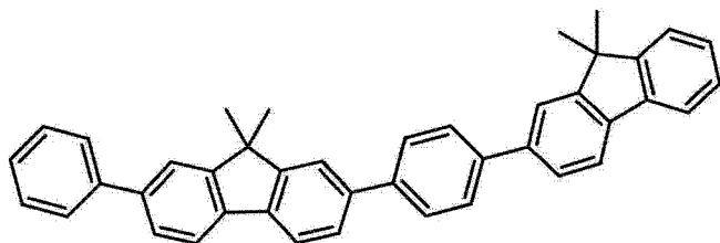
化合物 8
