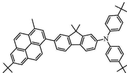
化合物 13
