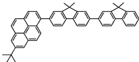
[0088] 化合物 6
