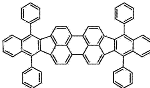
化合物 5
