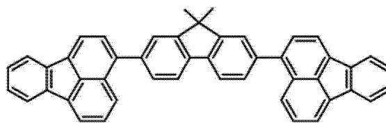
化合物 7
