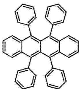
[0086] 化合物 4
