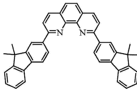
化合物 9
