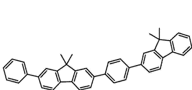
[0091] 化合物 8
