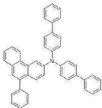
化学式 1-23
