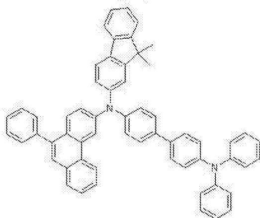
化学式 2-19
