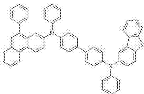
化学式 2-25
