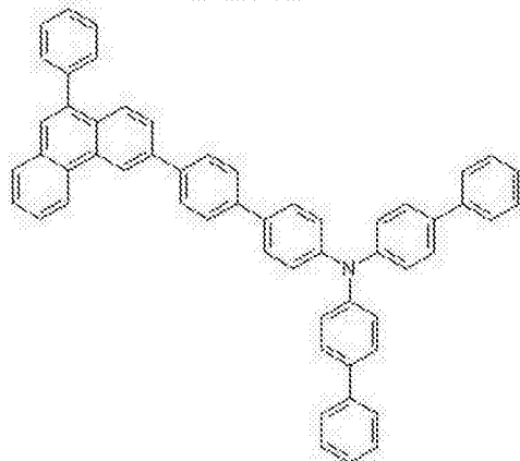
化学式 1-11
