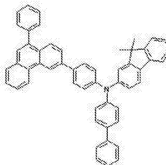
化学式 1-10
