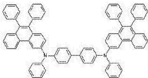
化学式 2-1
