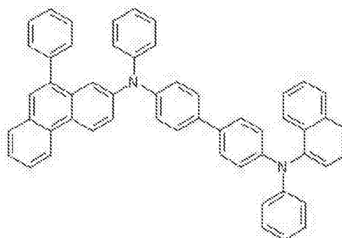
化学式 2-22
