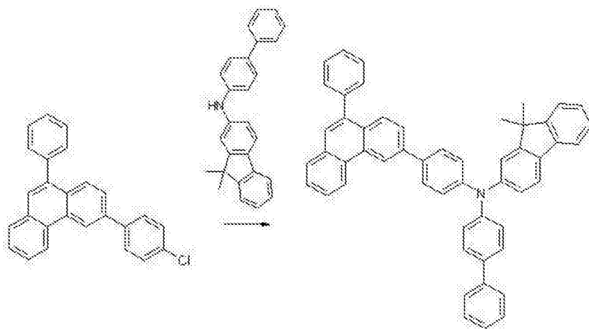
化学式 1-8
