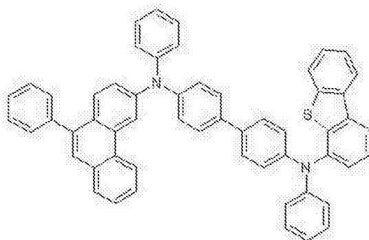
化学式 2-21
