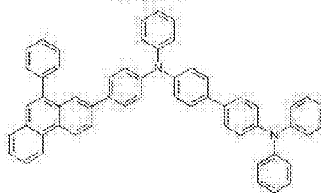
化学式 2-30
