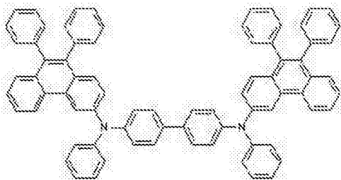
化学式 2-3
