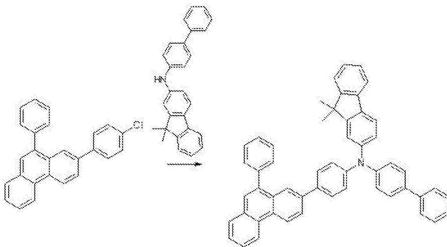
化学式 1-4
