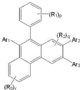
[化学式 1]
