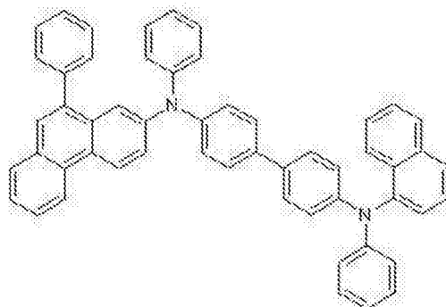
化学式 2-22
