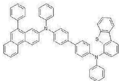
化学式 2-26
