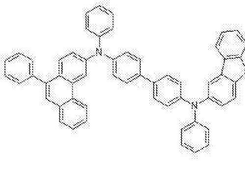
化学式 2-22
