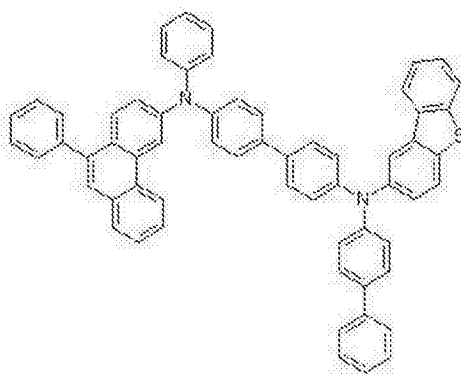
化学式 2-24
