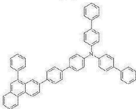
化学式 1-19
