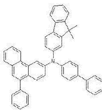
化学式 1-24
