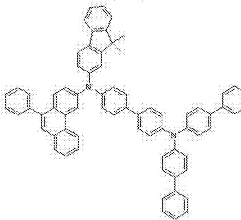
化学式 2-20
