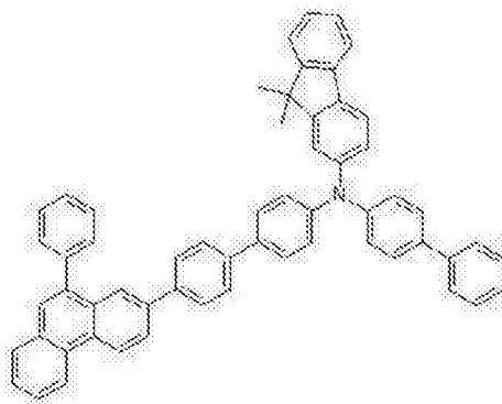
化学式 1-20
