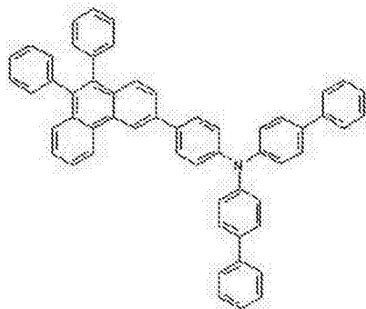
化学式 1-7
