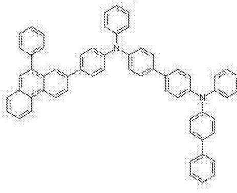
化学式 2-30
