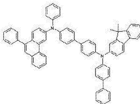
化学式 2-14
