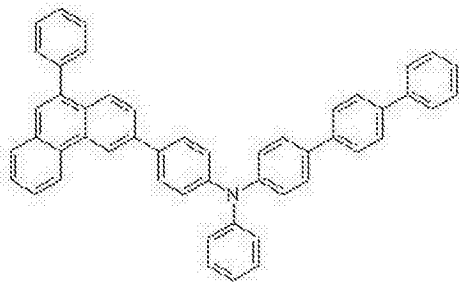
化学式 1-11
