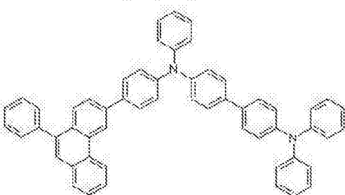
化学式 2-29
