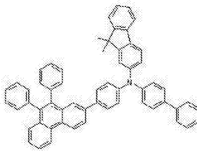
化学式 1-4
