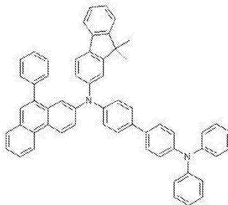
化学式 2-10
