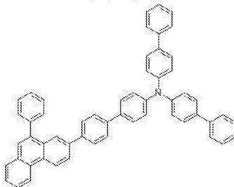
化学式 1-20
