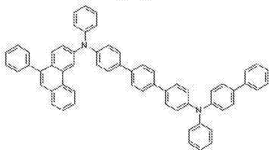
化学式 2-15
