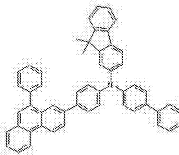
化学式 1-6
