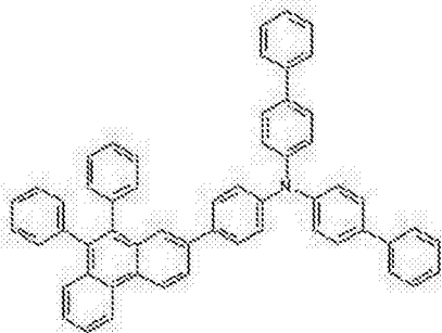
化学式 1-3
