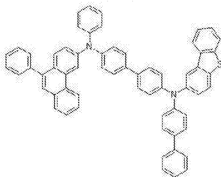
化学式 2-24
