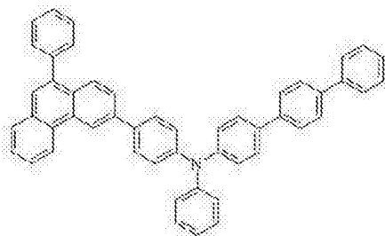
化学式 1-11
