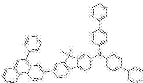
化学式 1-19
