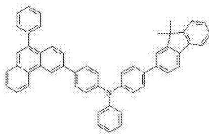
化学式 1-12
