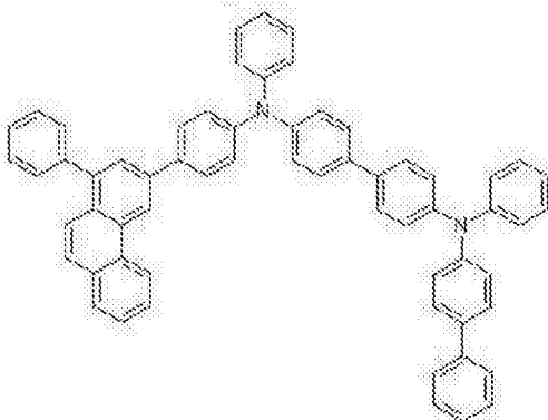
化学式 2-29
