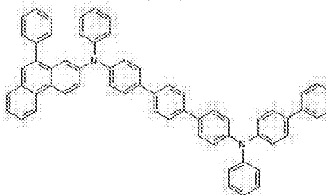
化学式 2-10
