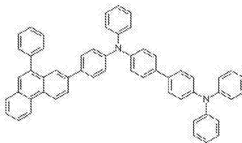
化学式 2-30
