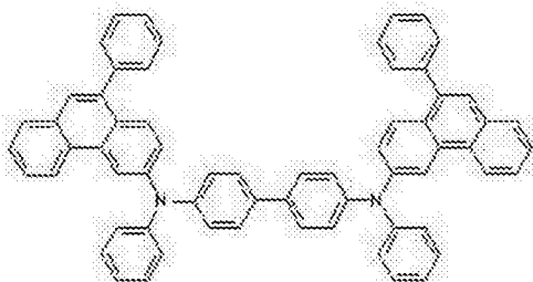
化学式 2-5
