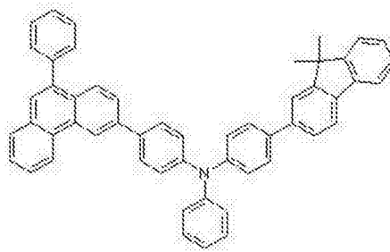
化学式 1-12
