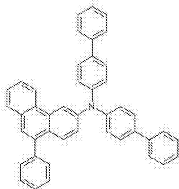
化学式 1-23
