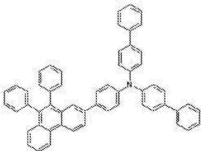
化学式 1-3
