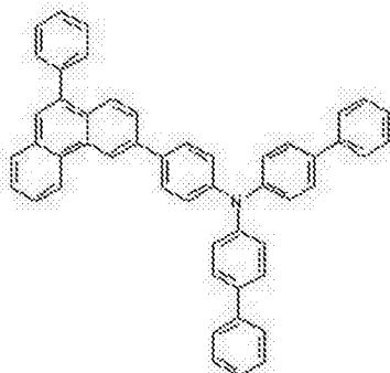
化学式 1-9
