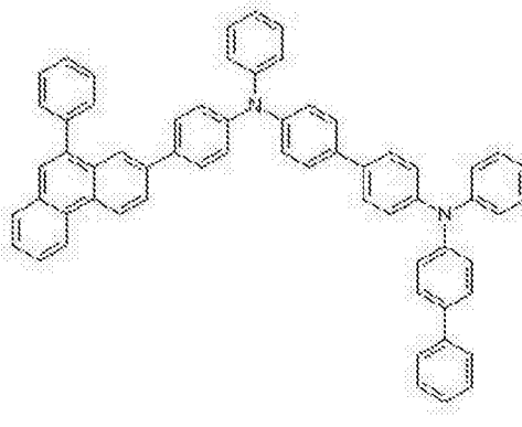
化学式 2-30
