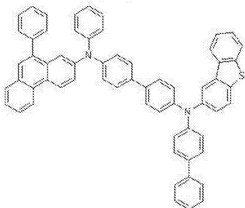
化学式 2-25
