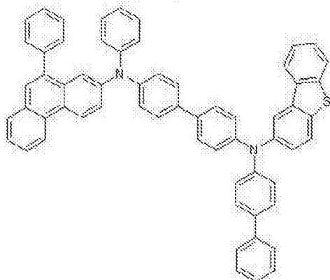
化学式 2-25
