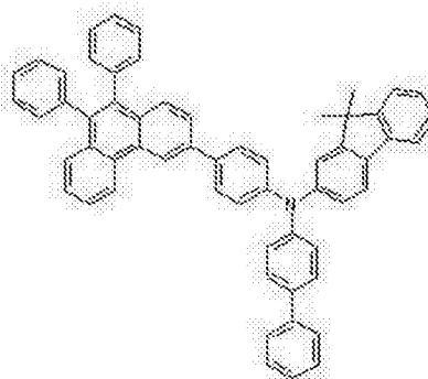
化学式 1-8
