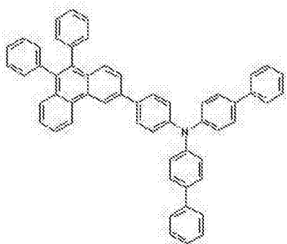
化学式 1-7
