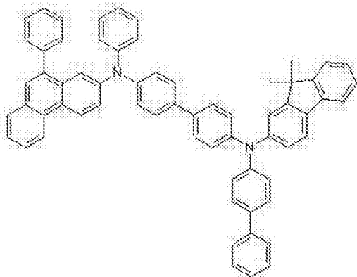
化学式 2-7
