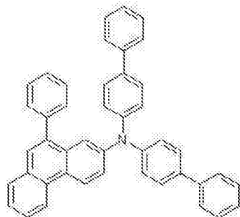
化学式 1-23
