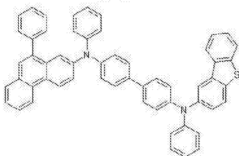
化学式 2-25
