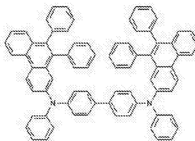
化学式 2-4
