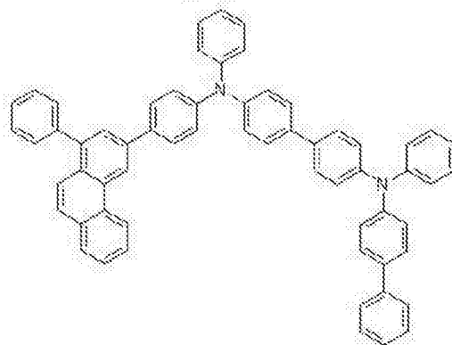
化学式 2-29
