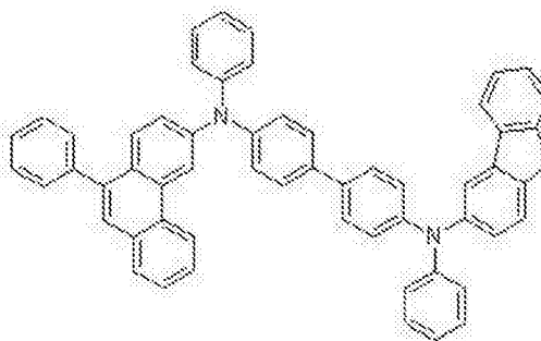
化学式 2-22
