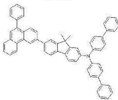
化学式 1-16
