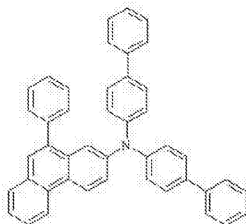
化学式 1-23
