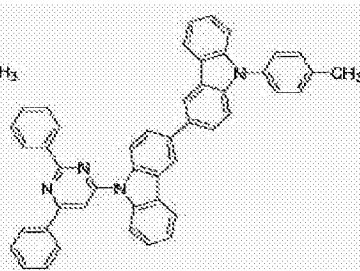
[化学式 B-209]
