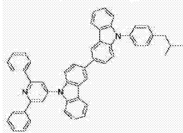
[化学式 A-113]
