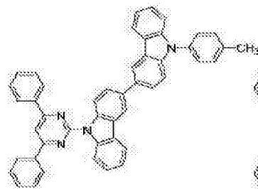
[化学式 B-205]
