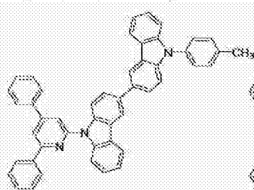
[化学式 A-108]
