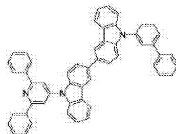
[化学式 A-115]
