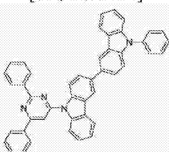
[化学式 B-205]
