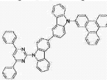
[化学式 B-220]
