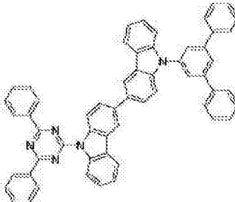
[化学式 B-110]
