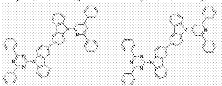
[化学式 B-110]
