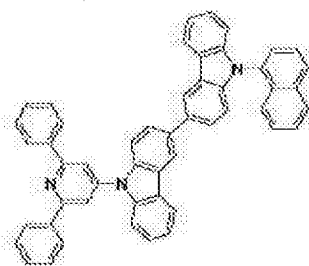
[化学式 A-119]
