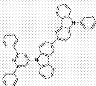
[化学式 A-105]
