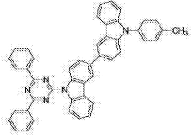
[化学式 B-106]
