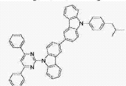
[化学式 B-212]
