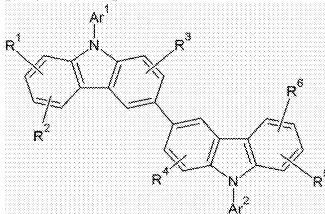
[化学通式 A-2]
