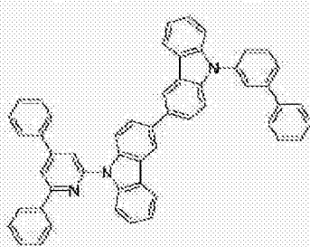
[化学式 A-114]
