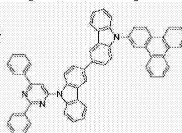
[化学式 B-221]
