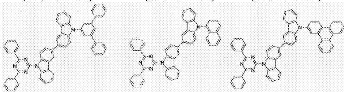
[化学式 B-110]
