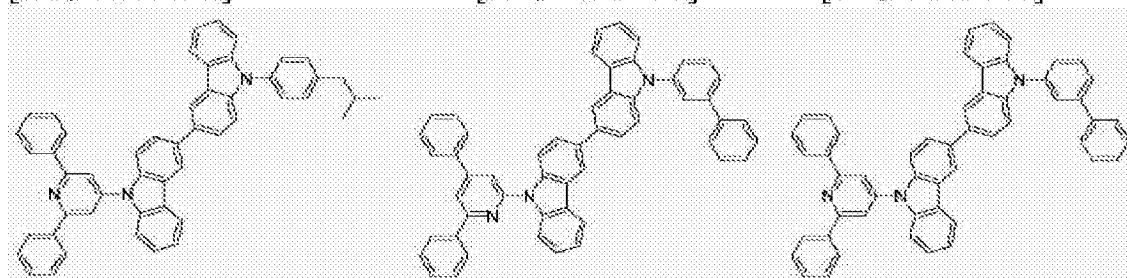
[化学式 A-113]
