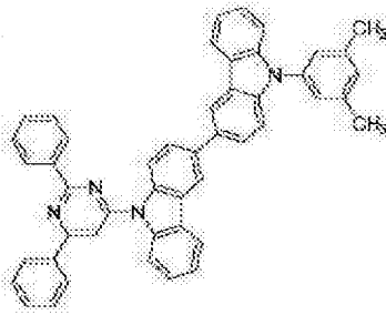
[化学式 B-211]
