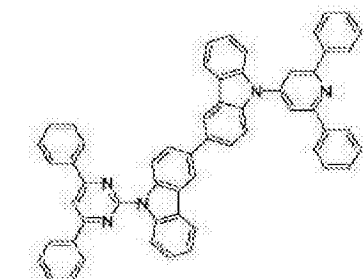
[化学式 B-220]
