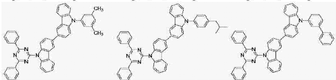
[化学式 B-107]
