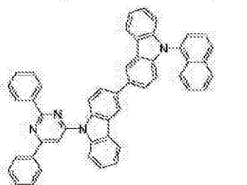
[化学式 B-219]
