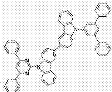
[化学式 B-216]
