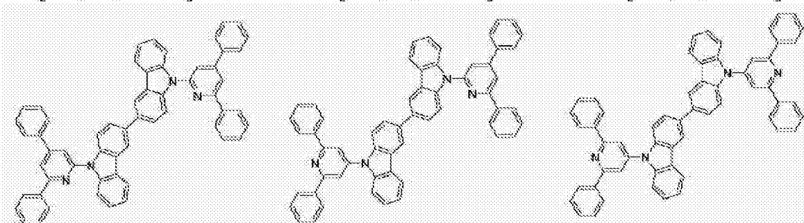
[化学式 A-119]
