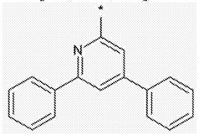
[化学通式 A-4]
