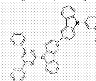
[化学式 B-214]
