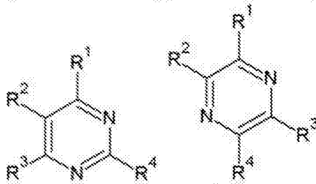
[化学通式 B-5] [化学通式 B-6]
