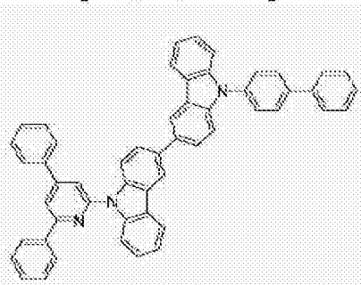
[化学式 A-106]
