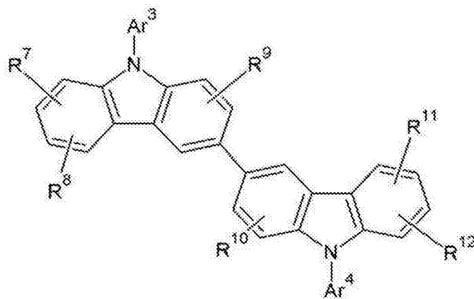
[化学通式 B-2]
