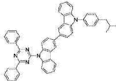
[化学式 B-108]
