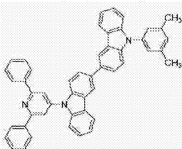
[化学式 A-111]
