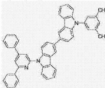
[化学式 A-110]
