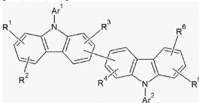
[化学通式 A-1]
