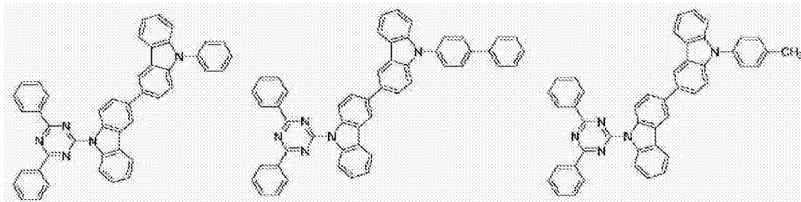
[化学式 B-104]
