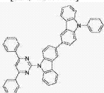
[化学式 B-204]
