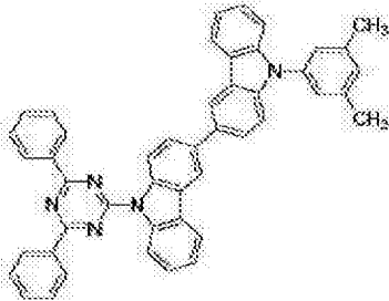
[化学式 B-107]
