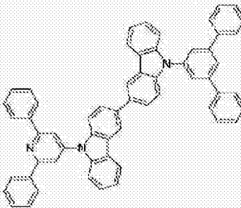
[化学式 A-117]
