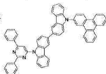
[化学式 B-221]
