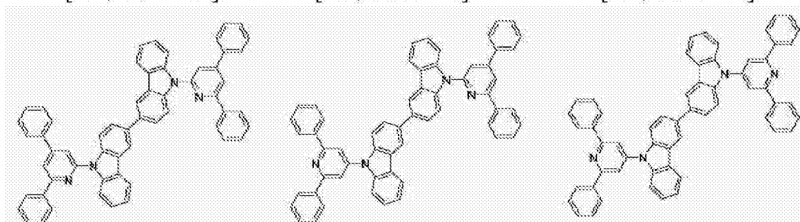
[化学式 A-119]
