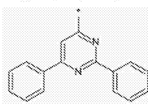
[化学式 B-9]
