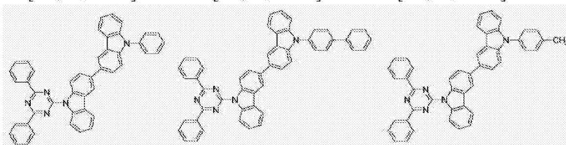
[化学式 B-104]
