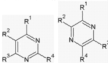
[化学通式 B-3] [化学通式 B-4]
