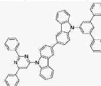
[化学式 B-217]
