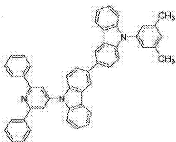
[化学式 A-111]
