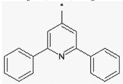
[化学通式 A-3]
