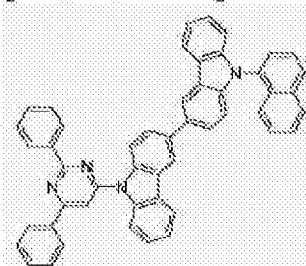
[化学式 B-219]
