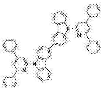
[化学通式 B-1]
