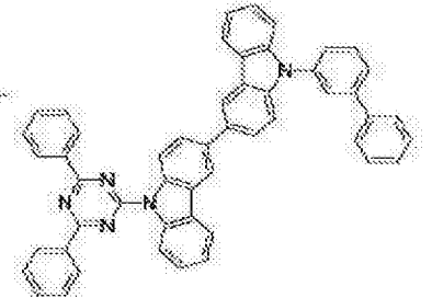
[化学式 B-109]
