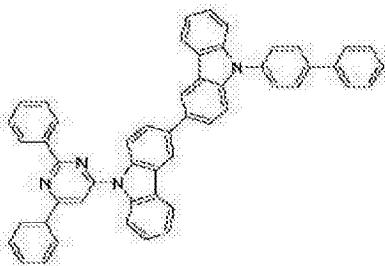
[化学式 B-204]
