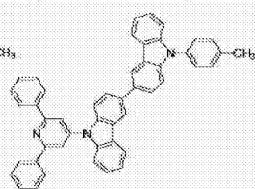
[化学式 A-109]
