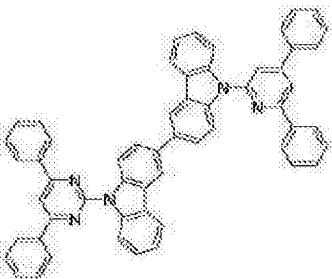
[化学式 B-219]
