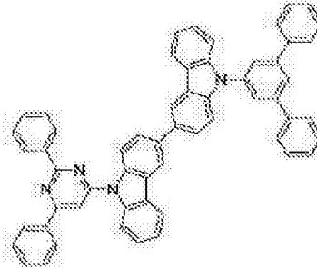
[化学式 B-217]
