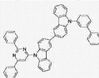
[化学式 B-215]
