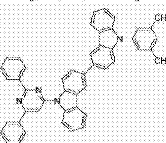
[化学式 B-211]
