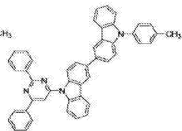
[化学式 B-206]
