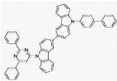
[化学式 B-207]
