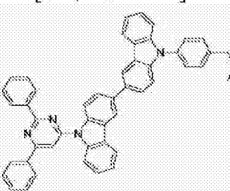
[化学式 B-213]
