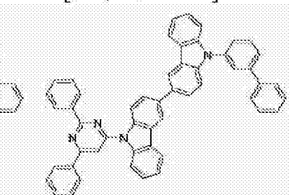
[化学式 B-215]
