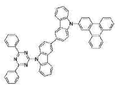
[化学式 B-109]
