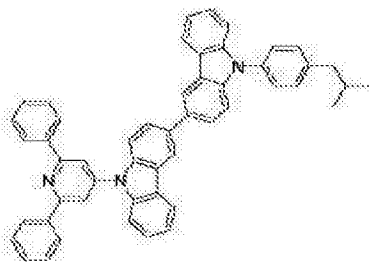
[化学式 A-113]
