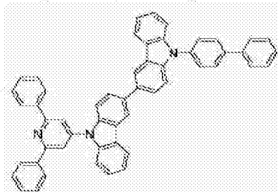
[化学式 A-107]
