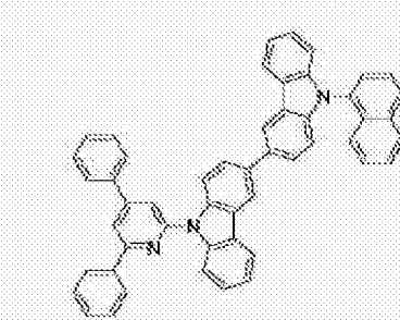
[化学式 A-118]
