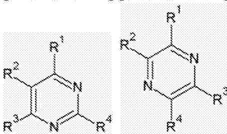
[化学通式 B-5] [化学通式 B-6]
