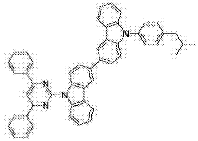
[化学式 B-212]
