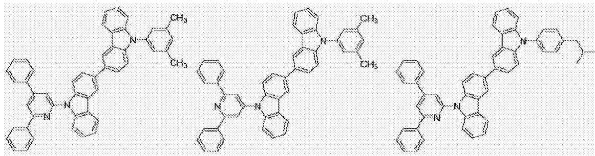
[化学式 A-110]
