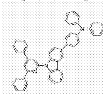
[化学式 A-104]
