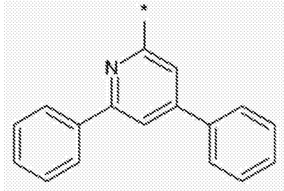
[化学通式 A-4]
