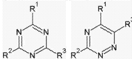
[化学通式 B-5] [化学通式 B-6]
