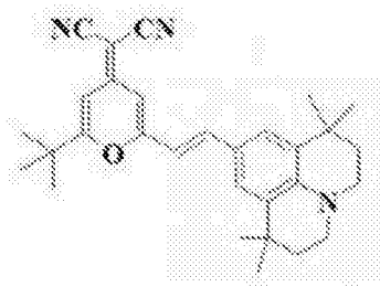
DCJTB(Propanedinitrile) ;
