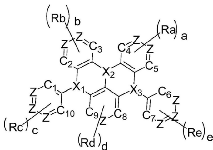
通式 (1)
