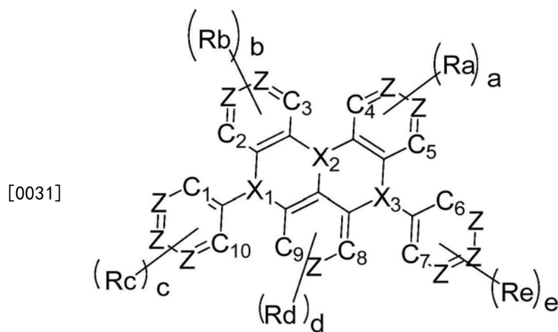
通式(1)
