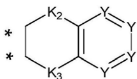
通式(4)
