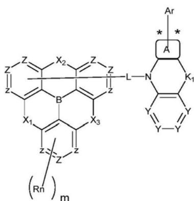
通式(3)
