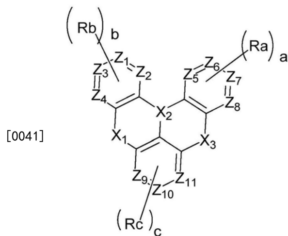
通式(2)
