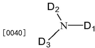
通式(17)
