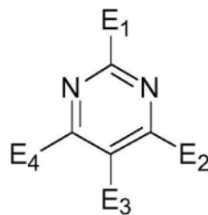
通式(21)
