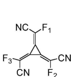
通式 (23)
