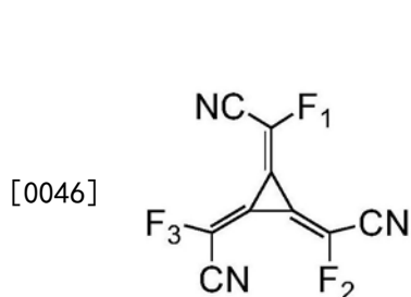
通式 (23)
