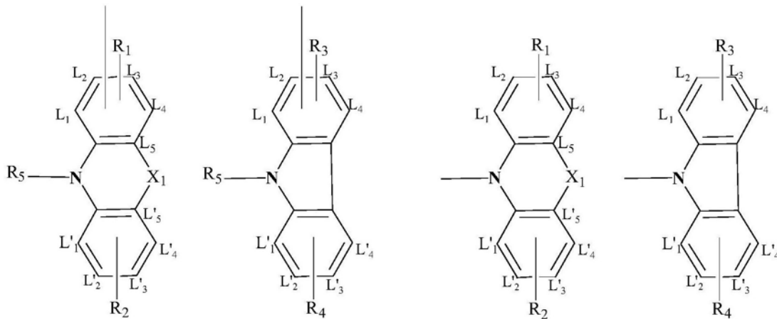
通式 (2)
