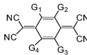
通式 (25)
