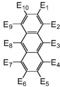
通式(18)
