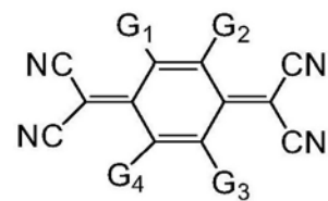
通式 (25)
