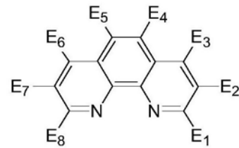
通式 (22)
