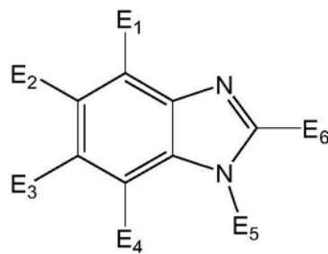
通式(19)
