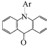
通式 (1)
