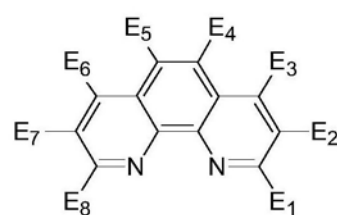
通式(22)
