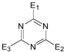
通式 (20)
