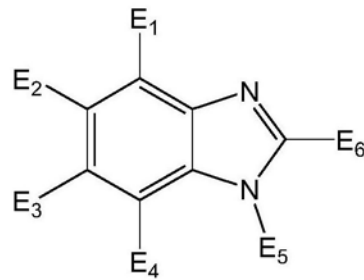
通式 (19)
