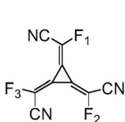
通式 (22)
