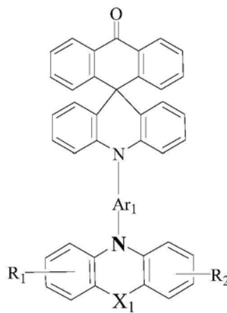
通式 (9)
