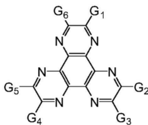
通式 (23)
