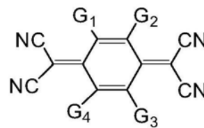
通式 (24)
