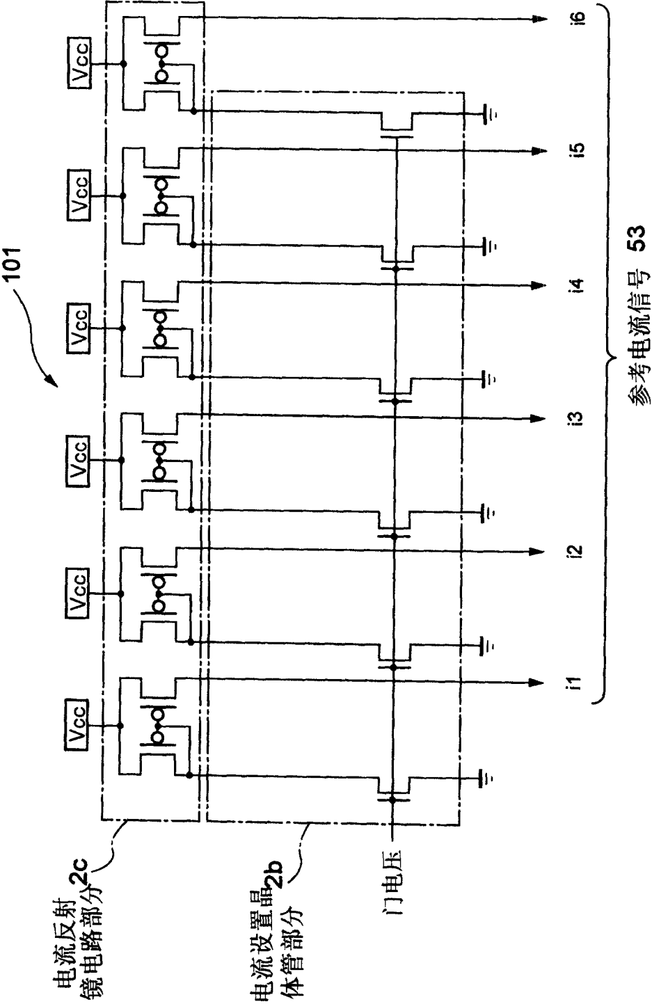
图14 现有技术
