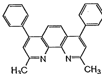
BCP
