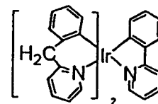
结构式 49
