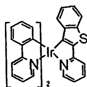
结构式 43
