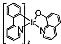
结构式 42
