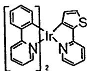
结构式 41
