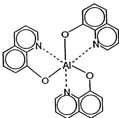
Alq3
