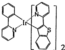
结构式 51
