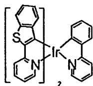
结构式 45
