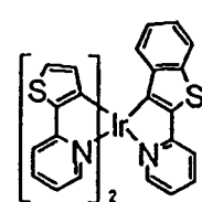
结构式 46
