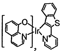
结构式 44
