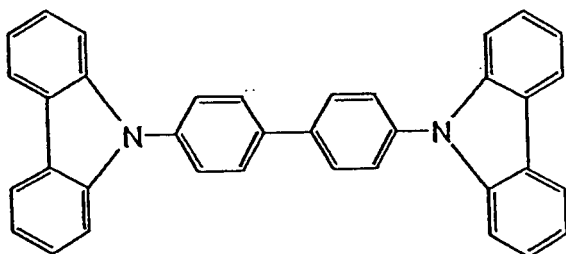
CBP
