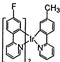
结构式 48
