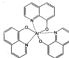
Alq3
