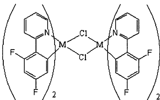
化学式III
