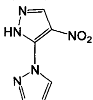
化合物 A'
