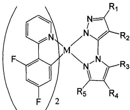
化学式I
