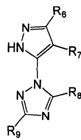
化学式V
