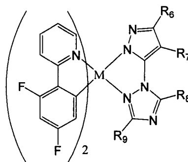
化学式II
