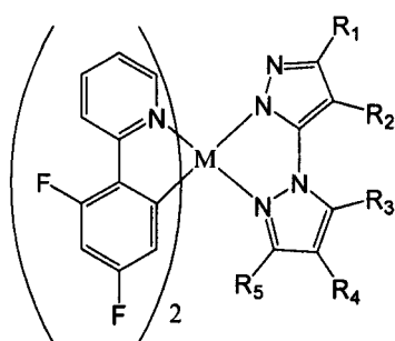
化学式I
