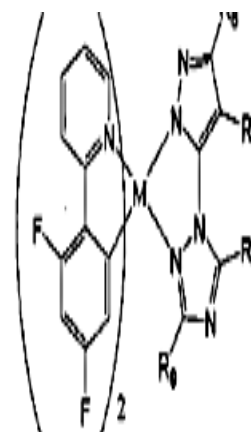
化学式II
