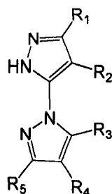
化学式IV
