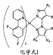
化学式I
