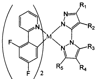
化学式I
