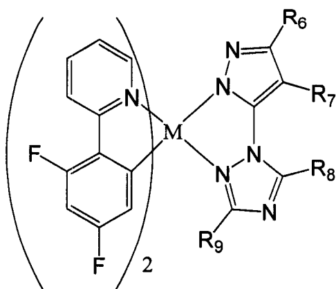
化学式II
