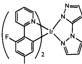
化合物 B 492 纳米
