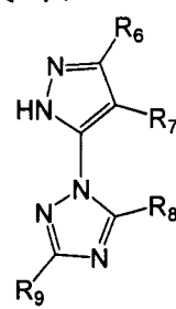
化学式V
