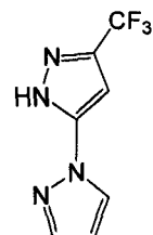
化合物 F'
