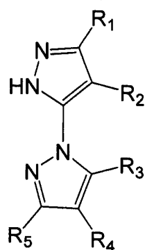
化学式IV
