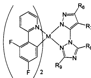
化学式II
