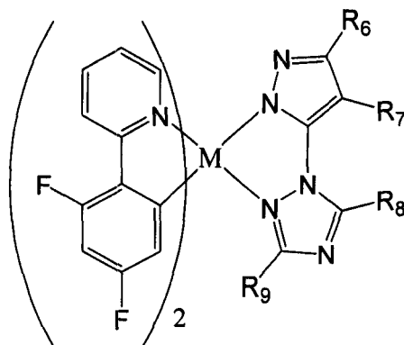
化学式II
