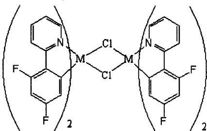
化学式III
