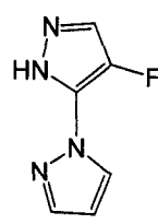
化合物 C'
