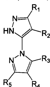
化学式IV
