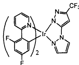
化合物 F
