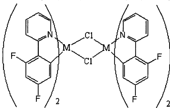
化学式III
