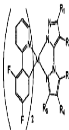
化学式I
