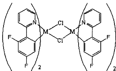
化学式III
