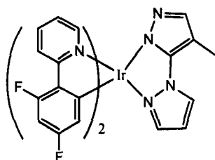
化合物 D 536 纳米
