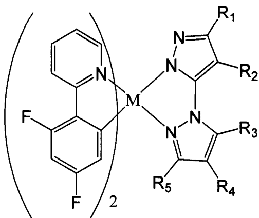
化学式I
