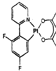
(4,6-F 2 ppy)Pt(acac)
