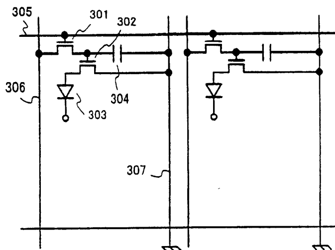
图 3 (现有技术)
