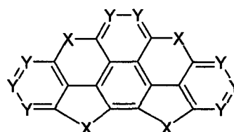
通式 (3)
