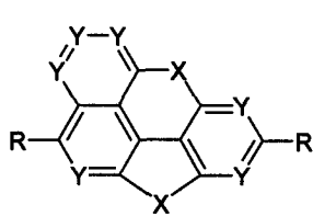
通式 (1a)
