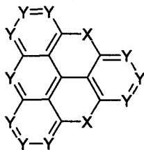
通式 (4)
