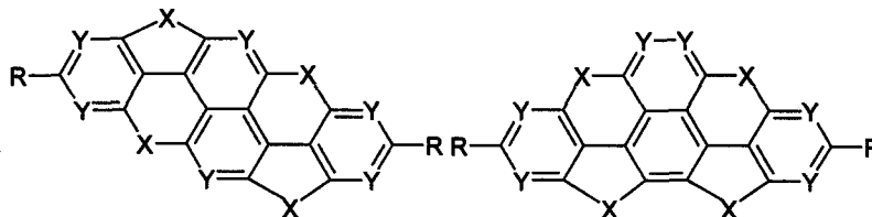
通式 (2a)
